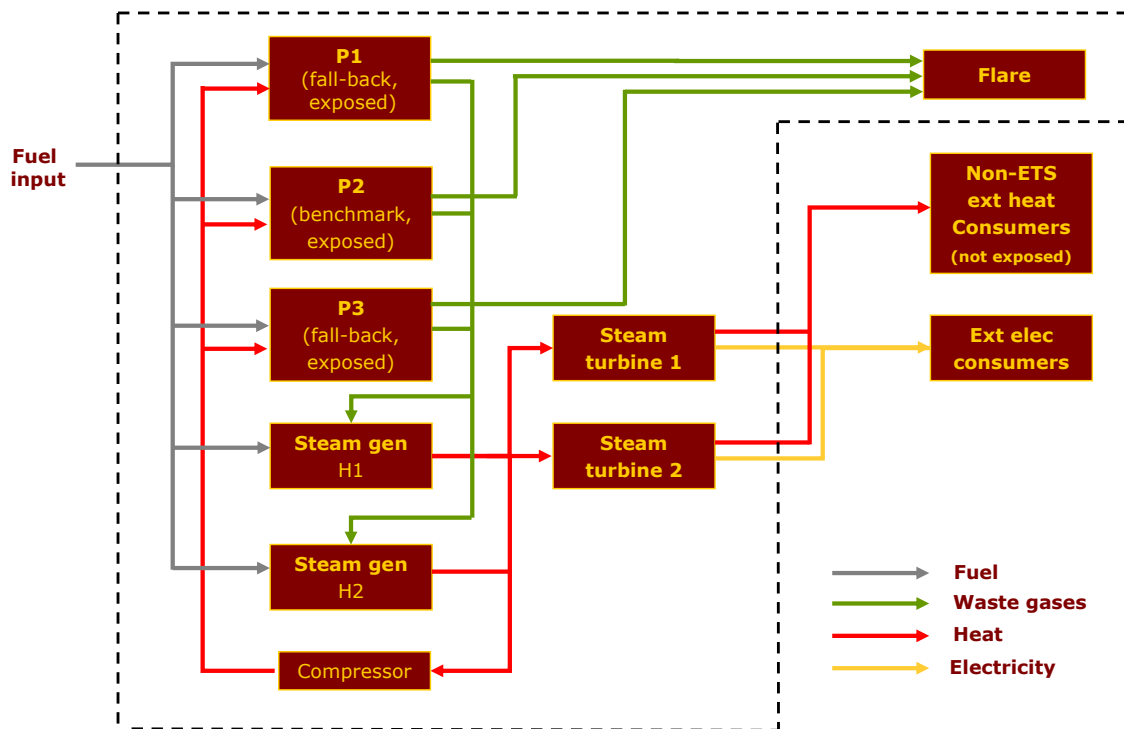
Slika 8 Primjer 1 - granice postrojenja; tokovi sirovina nisu prikazani (npr. ugljik koji se koristi kao redukcijski agens ili za kemijsku sintezu).
