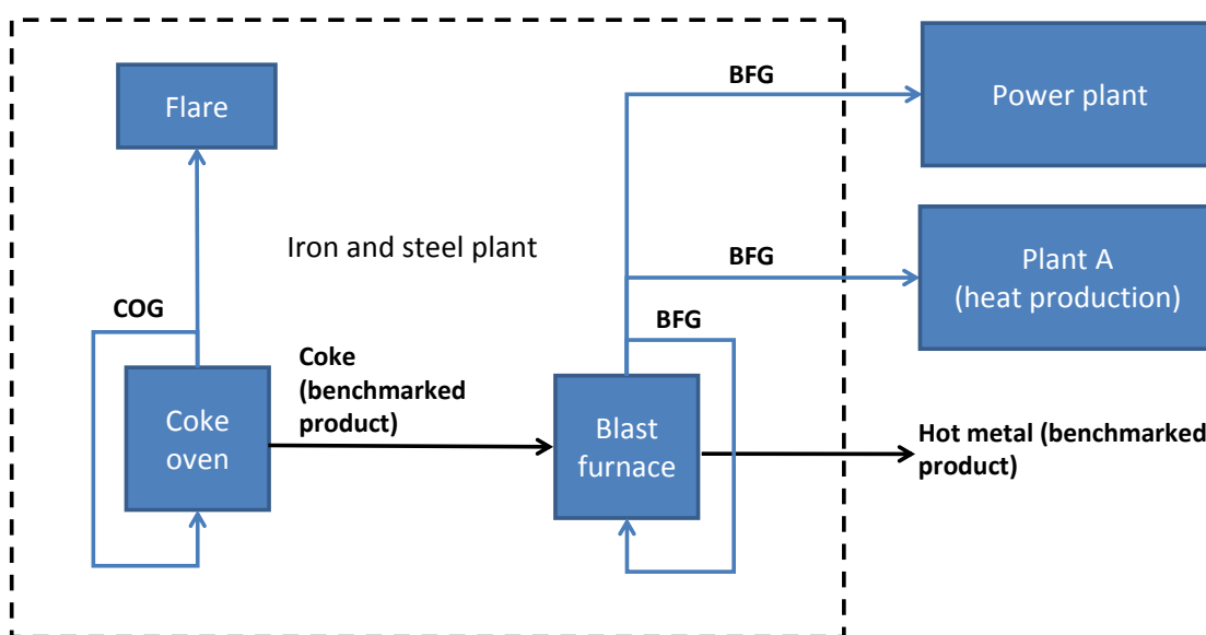
Slika 15 Primjer 2 - Otpadni plinovi nastali unutar granica referentnih vrijednosti proizvoda
