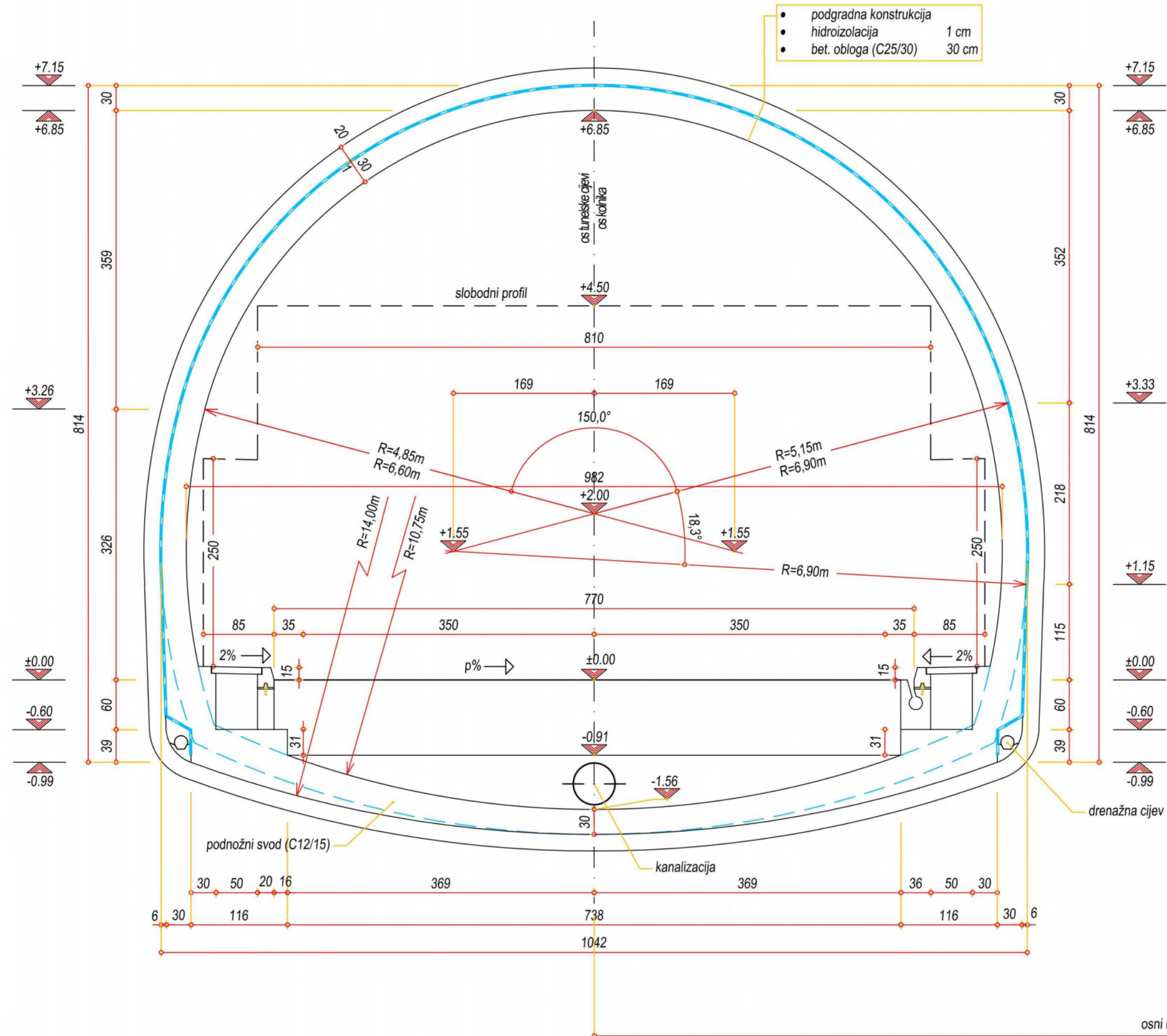
TUNELI "BOGAZ" I "LUŽNJAK" POPREČNI PRESJEK S PODNOŽNIM SVODOM 1:50
