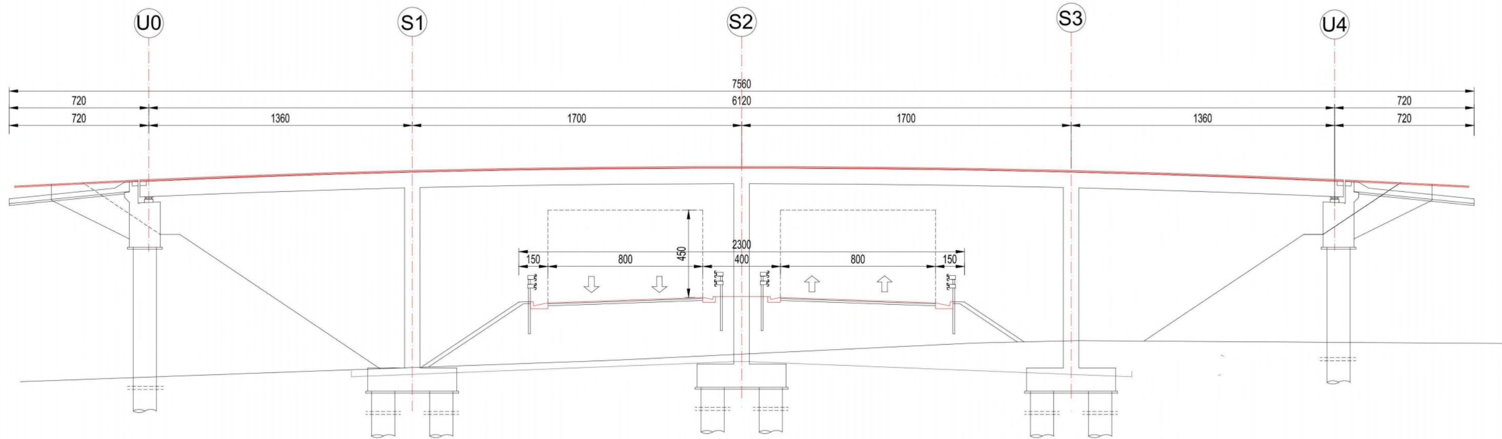
UZDUŽNI PRESJEK 1:200 - TIP 1
