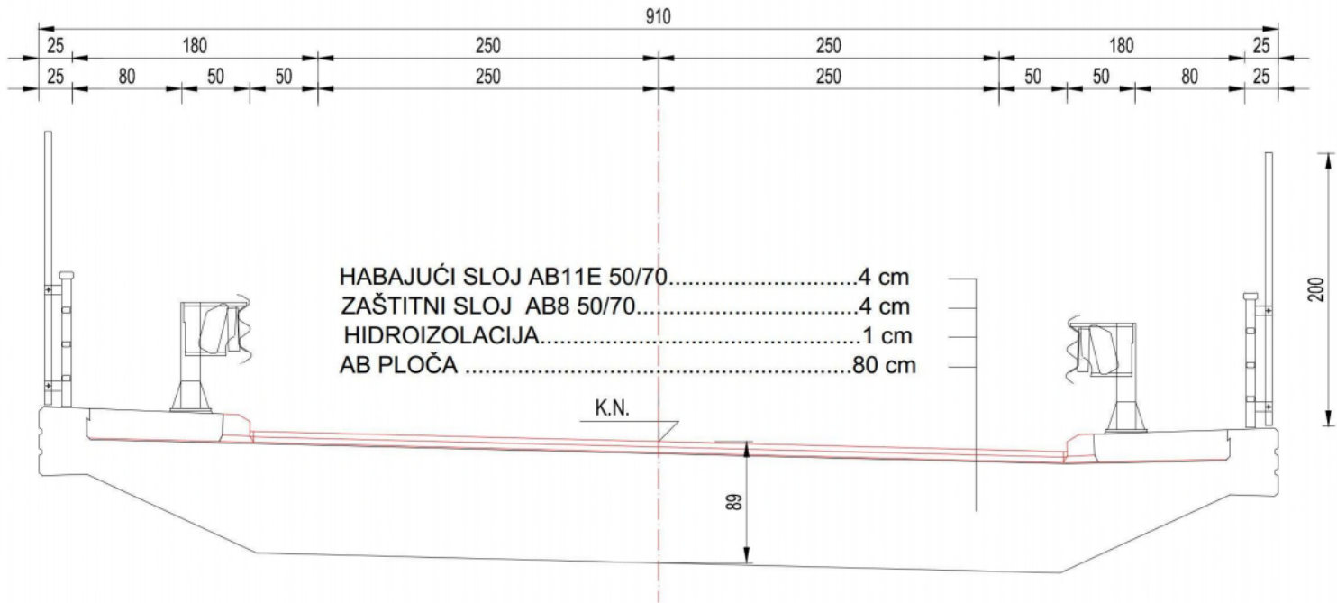
POPREČNI PRESJEK 1:50
