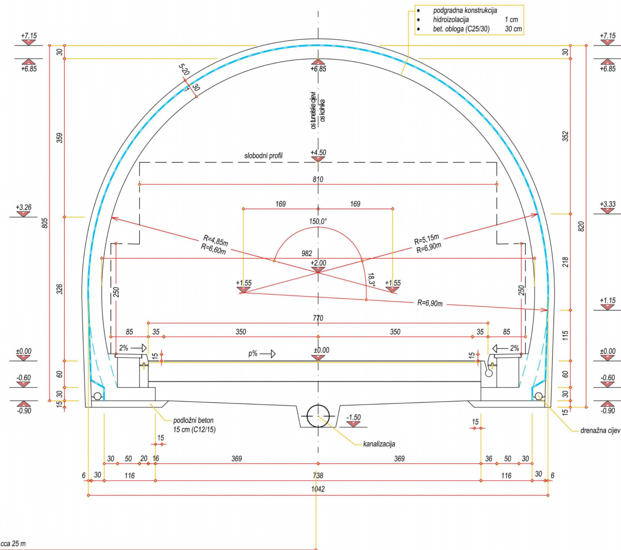
TUNELI "BOGAZ" I "LUŽNJAK" POPREČNI PRESJEK BEZ PODNOŽNOG SVODA 1:50
