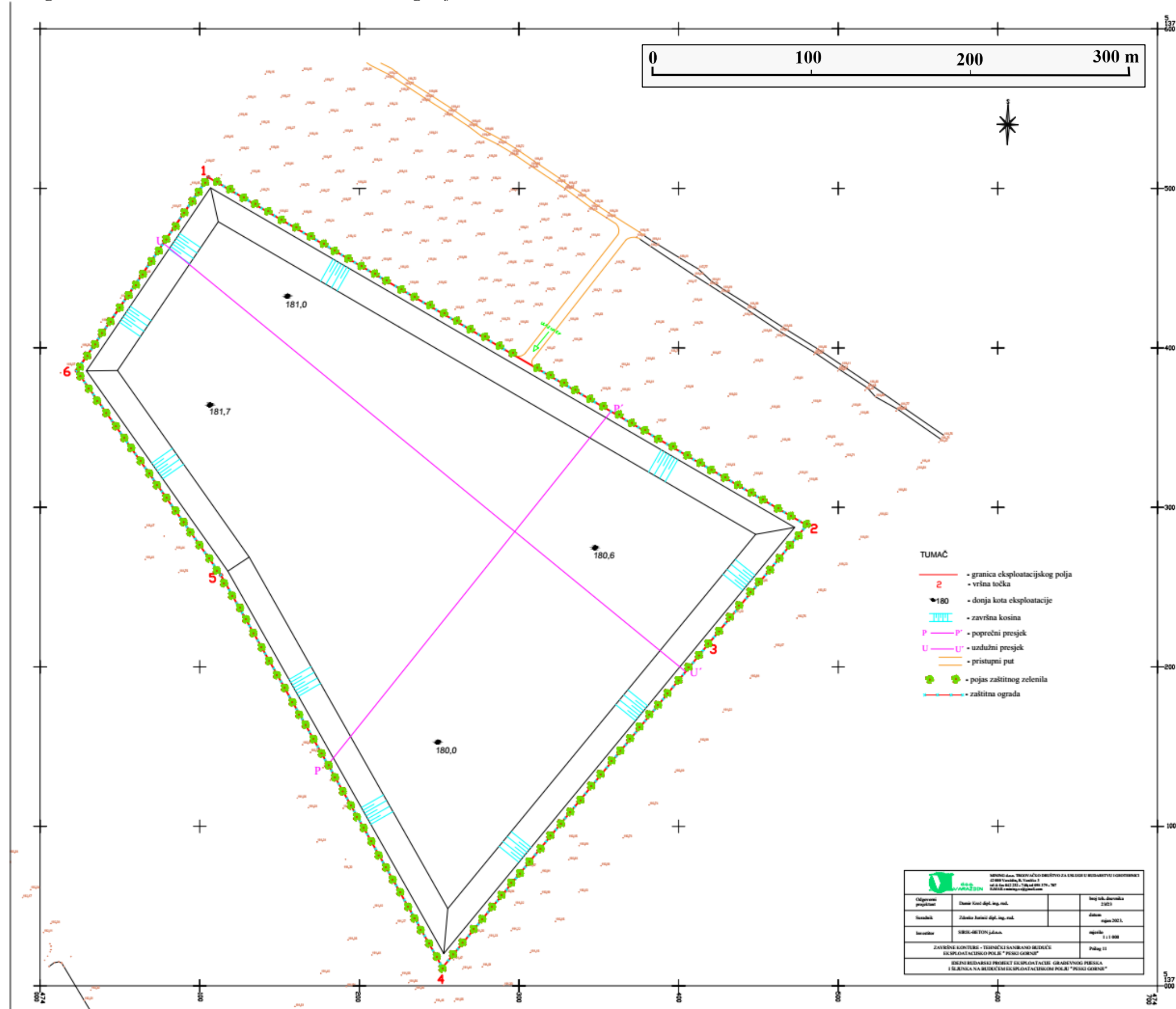
Prilog 4. Završne konture – tehnički sanirano EP „Peski gornji“
