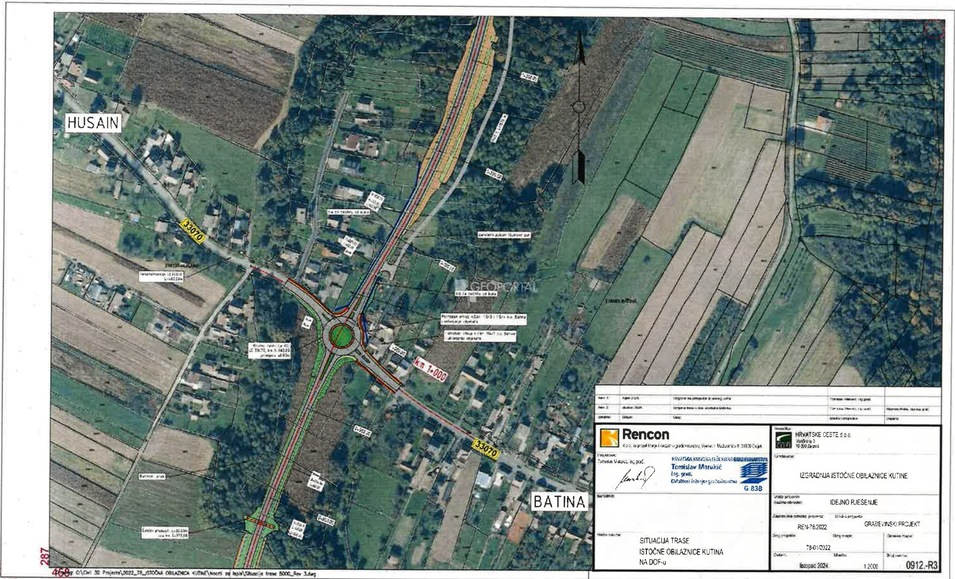
Prilog 2. Lokacije zida za zaštitu od buke
