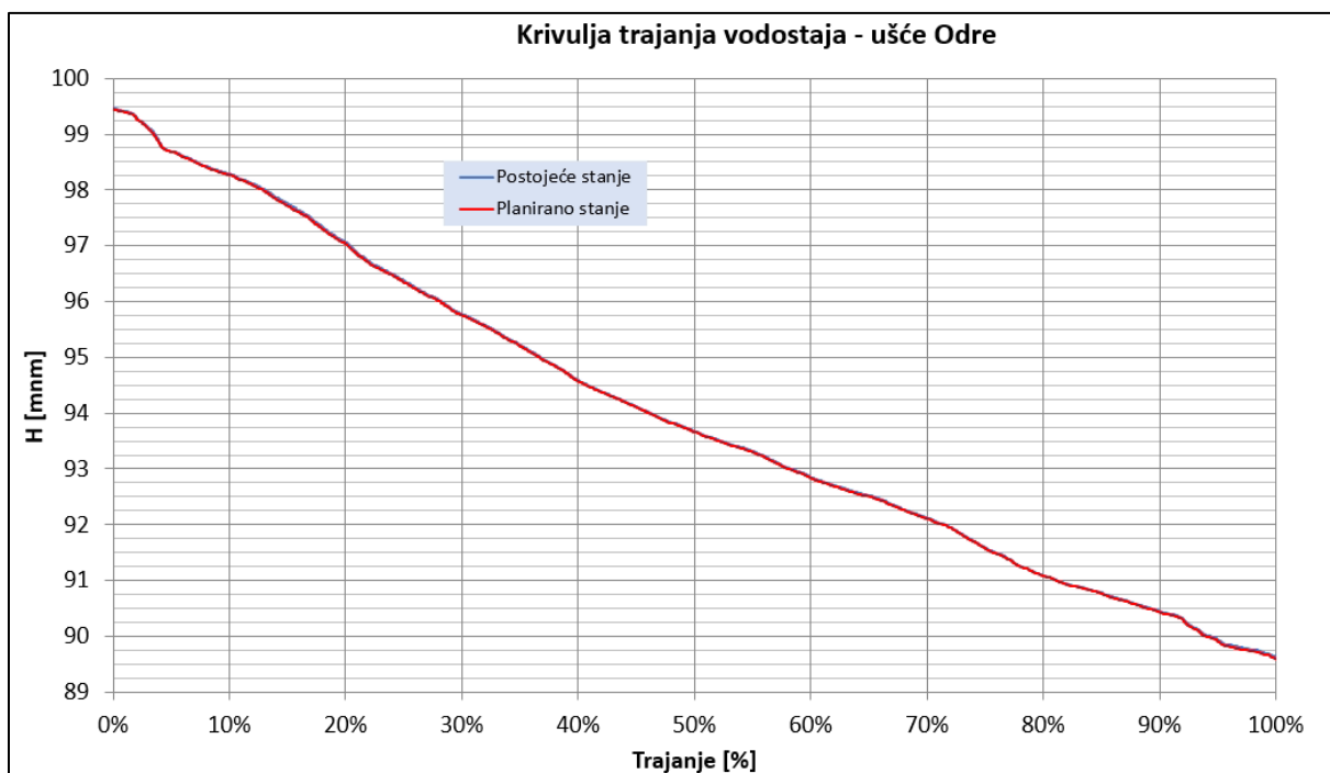
Slika 132. Krivulje trajanja vodostaja – ušće Odre, Kupa
