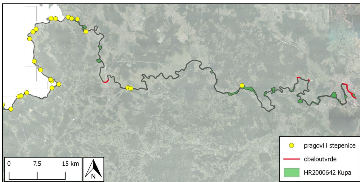
Slika 150. Postojeće obaloutvrde i pragovi/stepenice na rijeci Kupi
