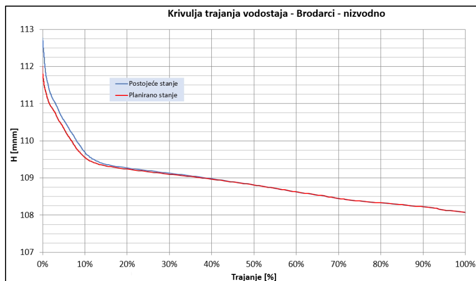
Slika 125. Krivulje trajanja vodostaja – Brodarci nizvodno, Kupa
