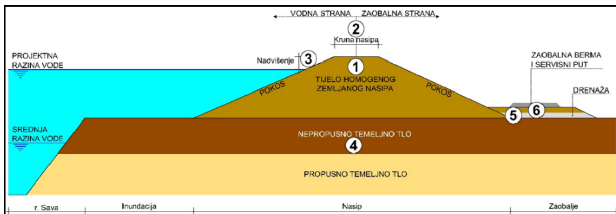
Slika 142. Modernizacija lijevoobalnih savskih nasipa – karakteristični presjek
