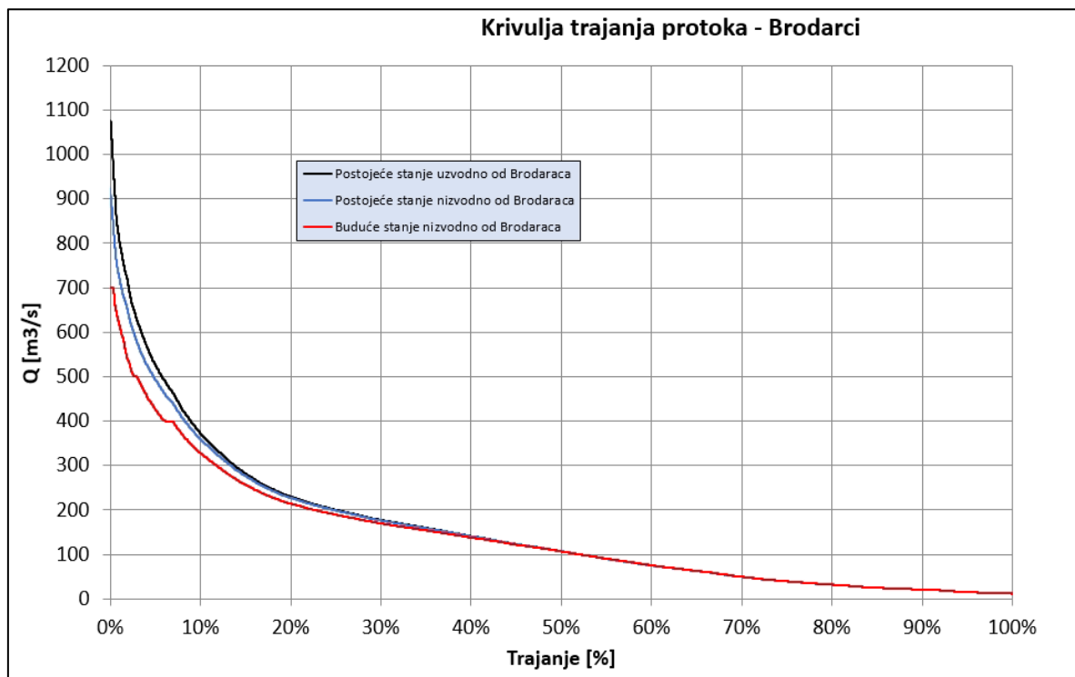
Slika 122. Krivulje trajanja protoka – Brodarci, Kupa
