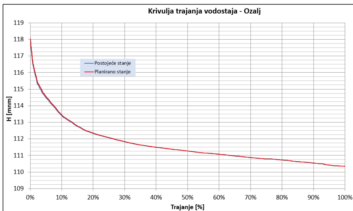
Slika 134. Krivulje trajanja vodostaja – DV Ozalj, Kupa
