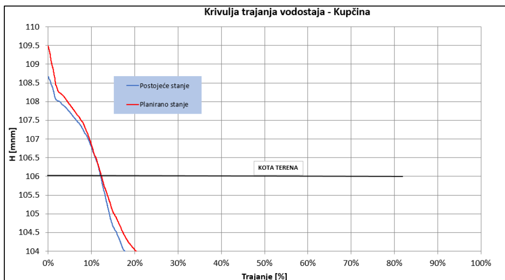
Slika 127. Krivulje trajanja vodostaja – retencija Kupčina
