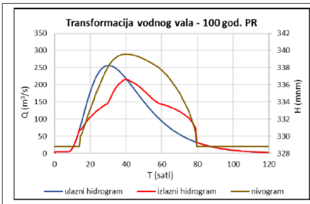
Slika 140. Transformacija vodnog vala kroz retenciju Ogulin za PP 100
