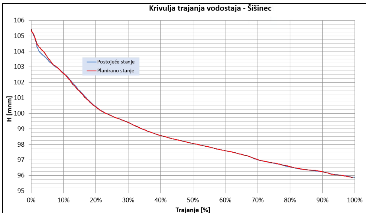
Slika 130. Krivulje trajanja vodostaja – VP Šišinec, Kupa
