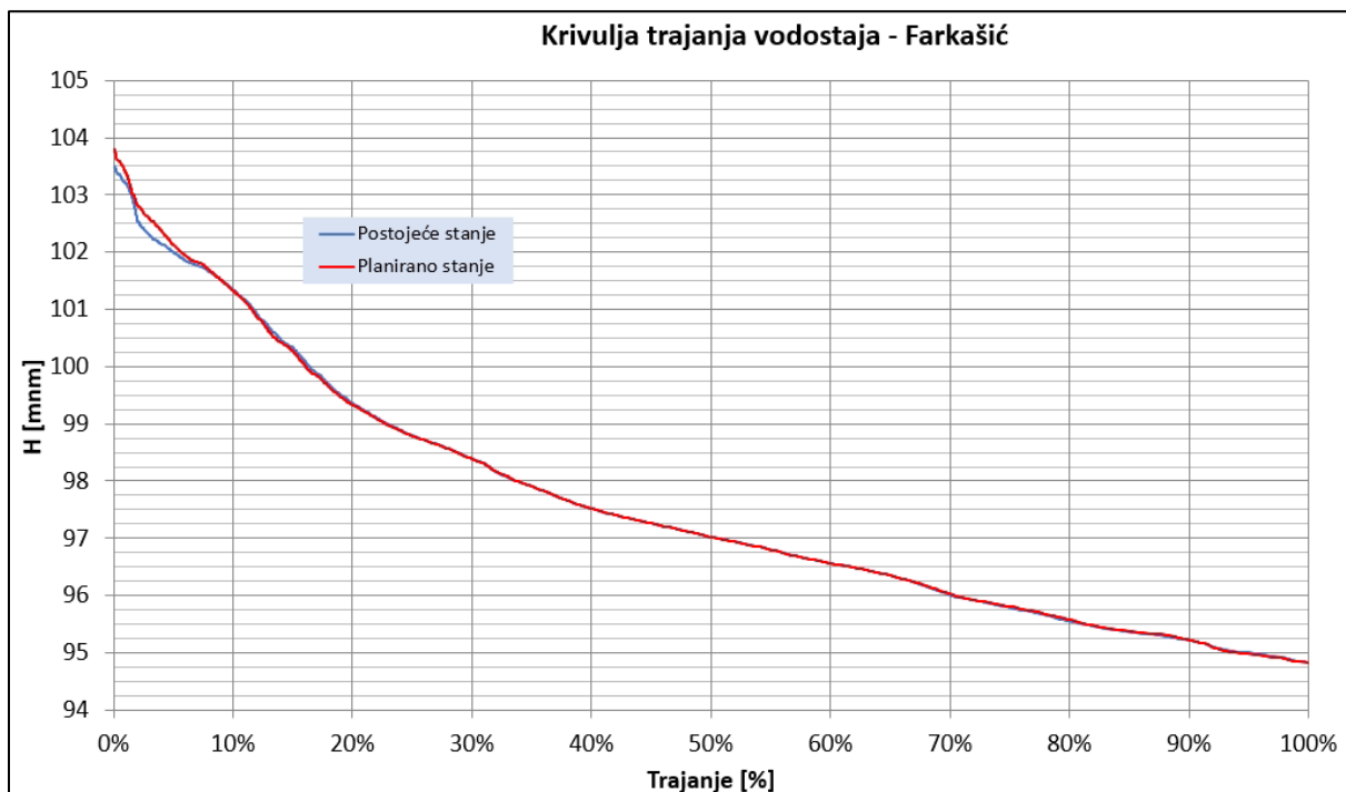
Slika 131. Krivulje trajanja vodostaja – VP Farkašić, Kupa
