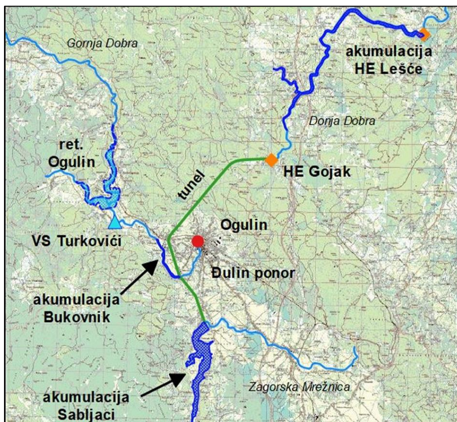
Slika 138. Situacijski prikaz ogulinskog sustava zaštite od poplava
