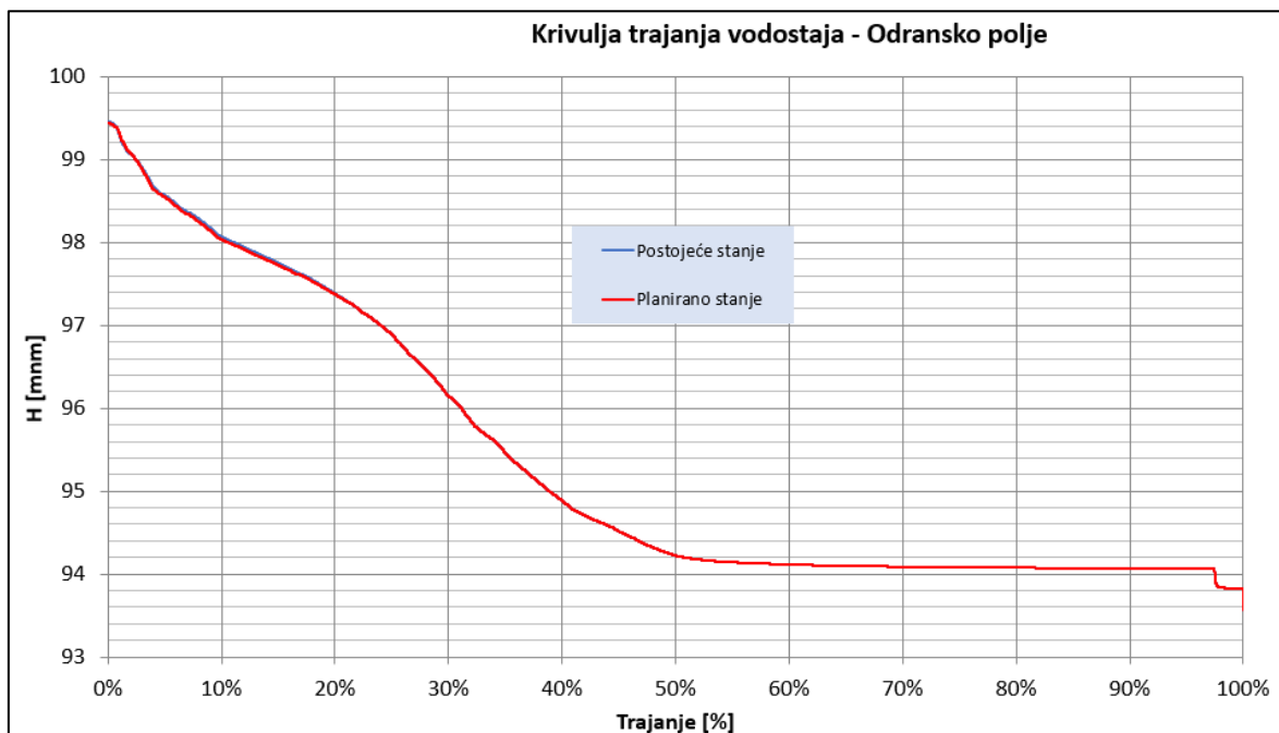
Slika 133. Krivulja trajanja vodostaja – Odransko polje
