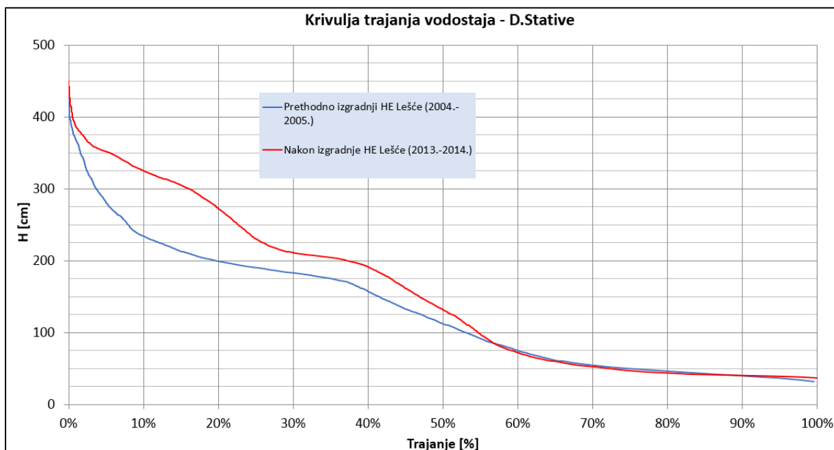
Slika 153. Krivulja trajanja vodostaja – D. Stative
