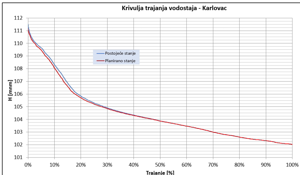
Slika 126. Krivulje trajanja vodostaja – VP Karlovac, Kupa
