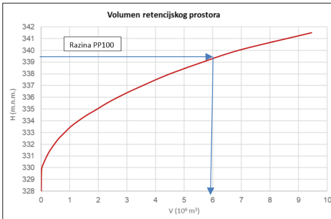
Slika 139. Volumetrijska krivulja retencije Ogulin
