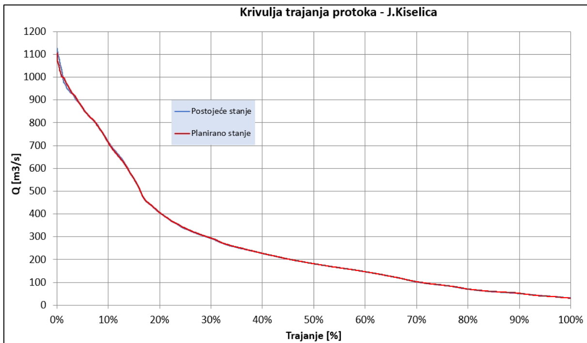
Slika 129. Krivulje trajanja protoka – VP J. Kiselica, Kupa
