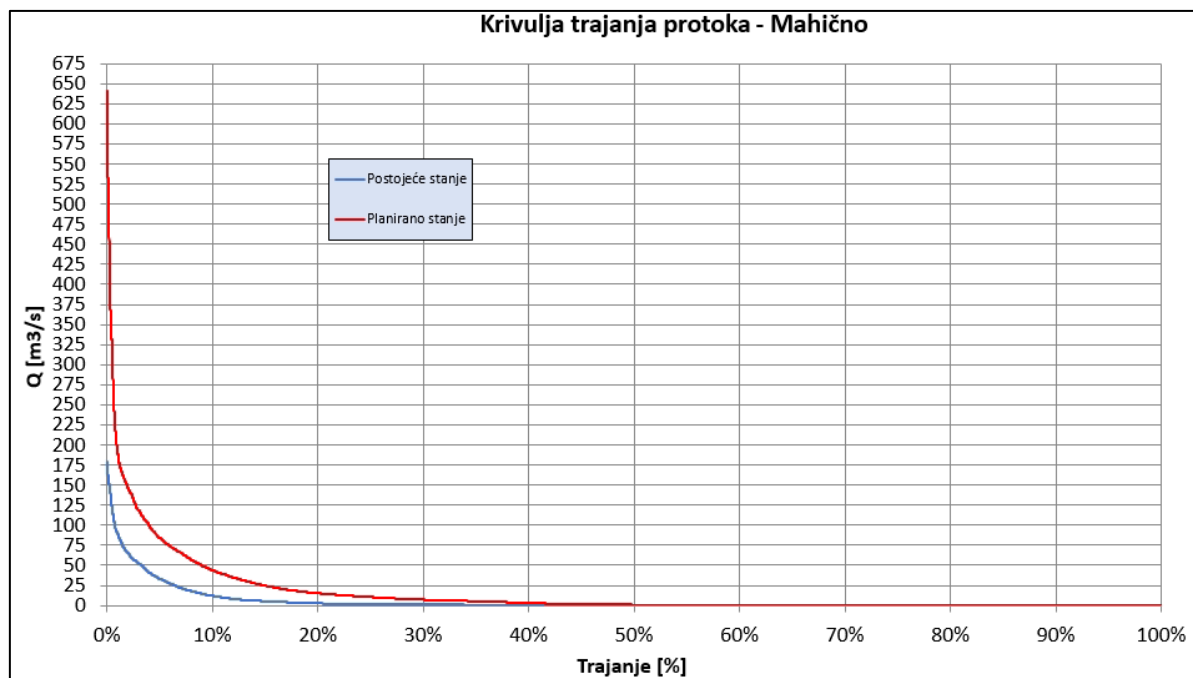
Slika 123. Krivulje trajanja protoka – VP Mahično, kanal Kupa-Kupa
