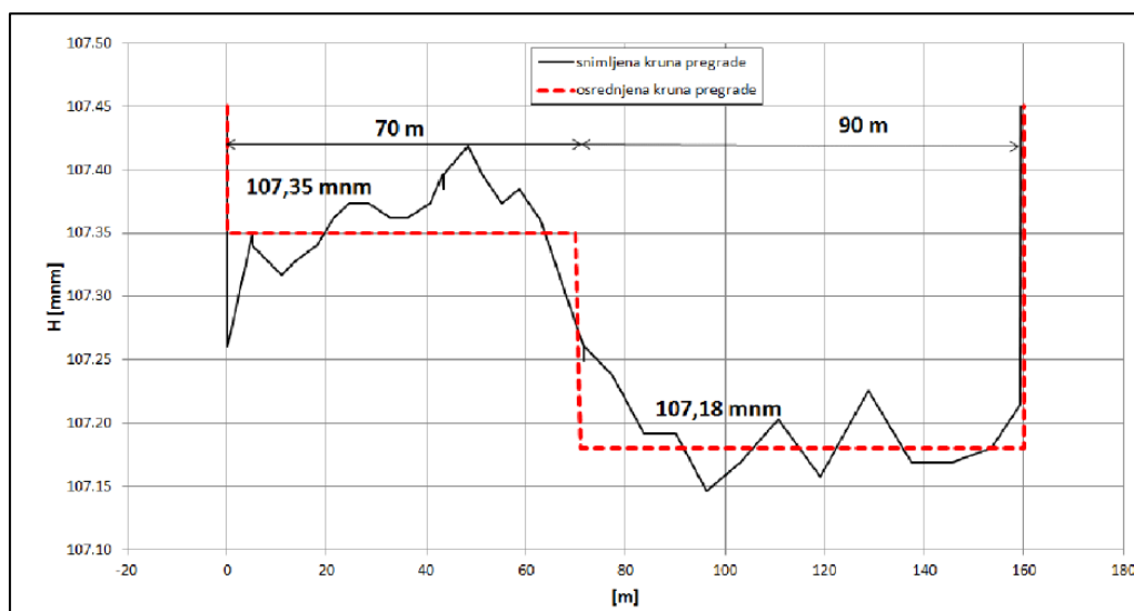
Slika 149. Profil brane na lokaciji zahvata MHE Korana 1
