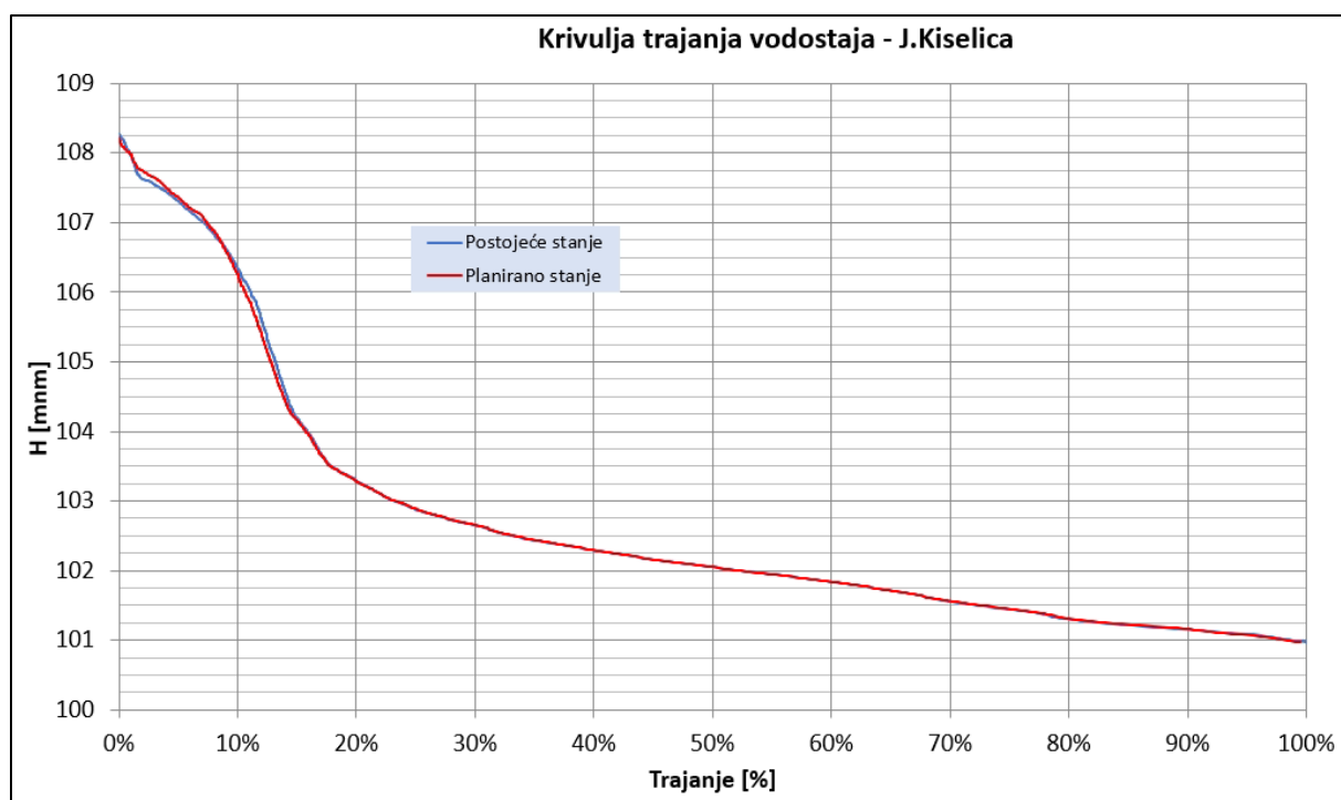
Slika 128. Krivulje trajanja vodostaja – VP J. Kiselica, Kupa
