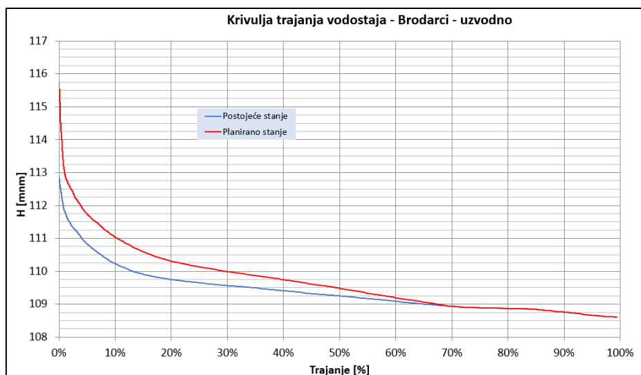
Slika 124. Krivulje trajanja vodostaja – Brodarci uzvodno, Kupa
