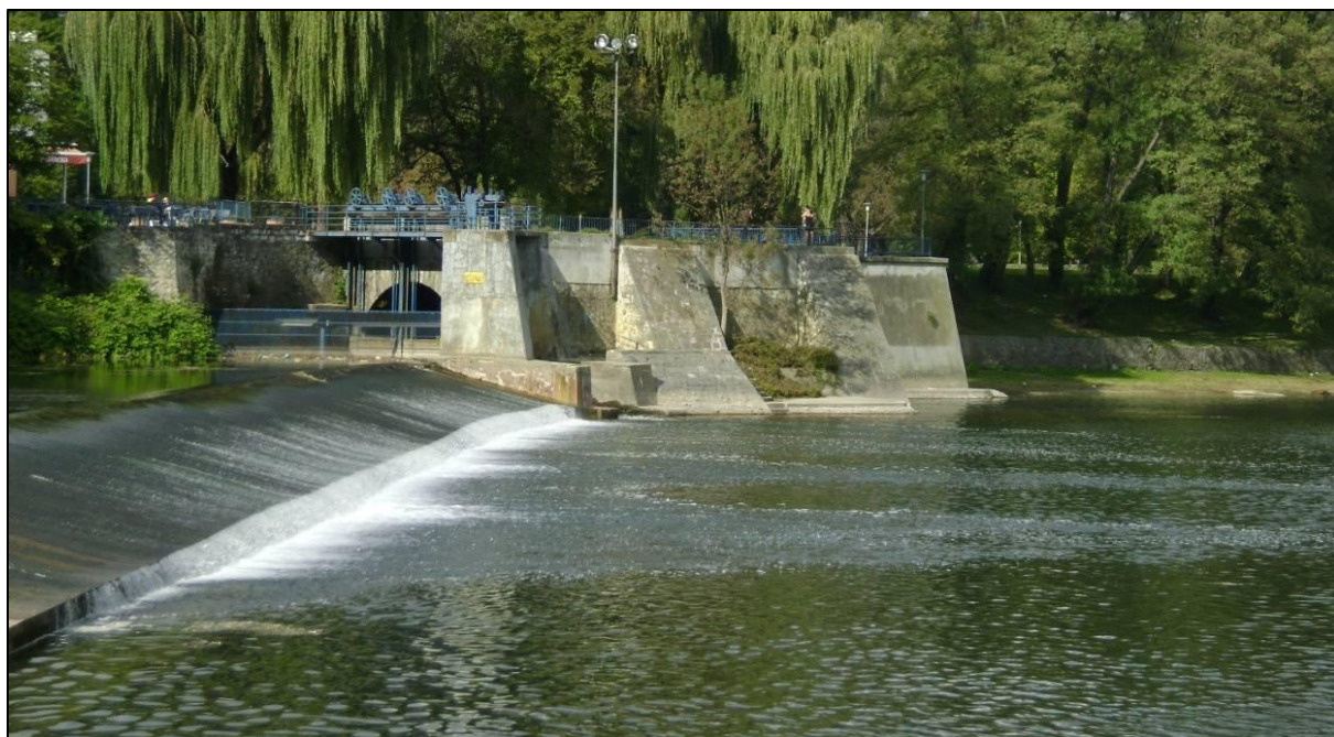
Slika 148. Postojeća brana na lokaciji zahvata MHE Korana 1
