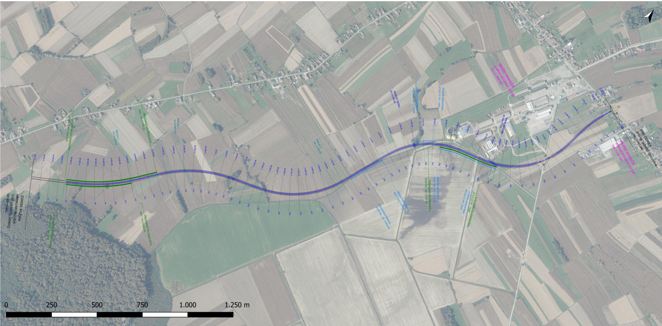
Grafički prikaz A-5 Situacija planirane prometnice na ortofoto podlozi
