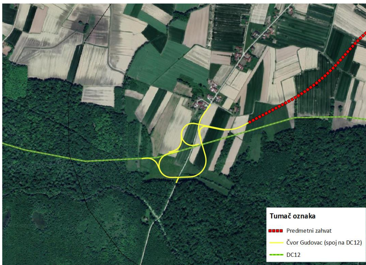
Grafički prikaz D-10: Spoj na buduću DC12 preko čvora Gudovac
