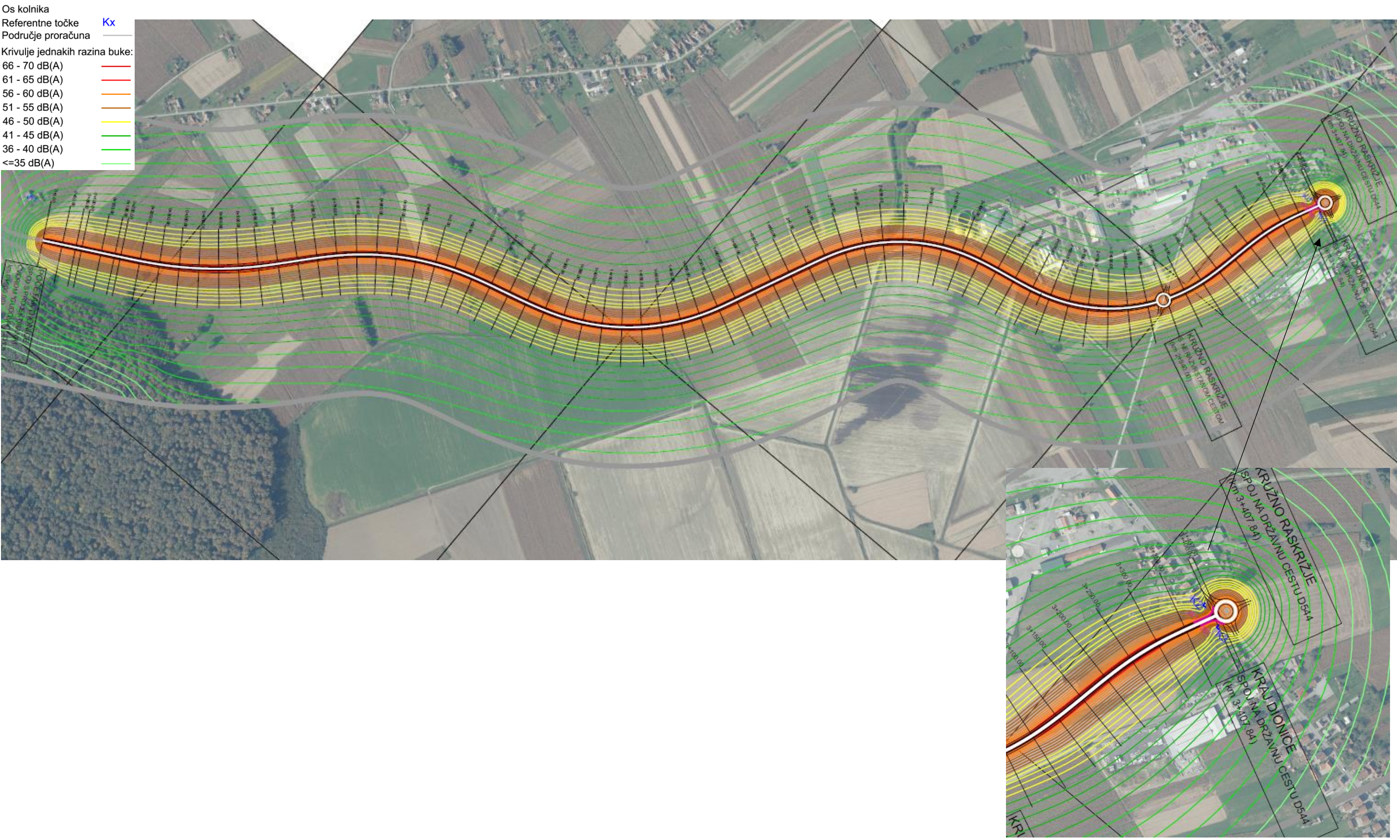
Grafički prikaz D-7: Prikaz širenja buke u okoliš – noćno razdoblje – situacija nakon postavljanja zidova za zaštitu od buke
