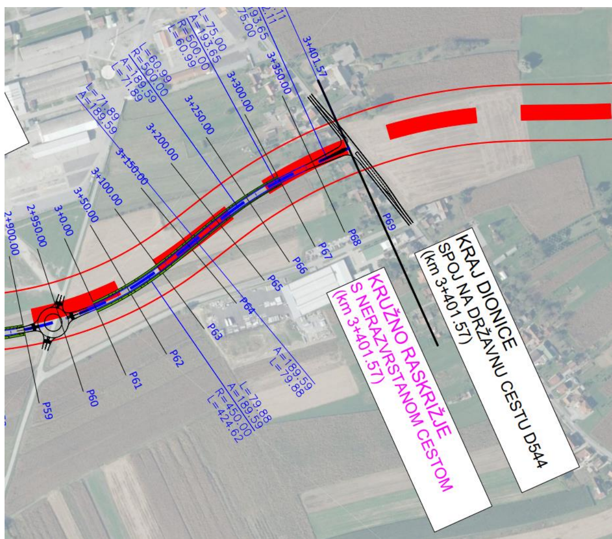
Grafički prikaz B-2: Spoj s državnom cestom DC544 – Varijanta 1
