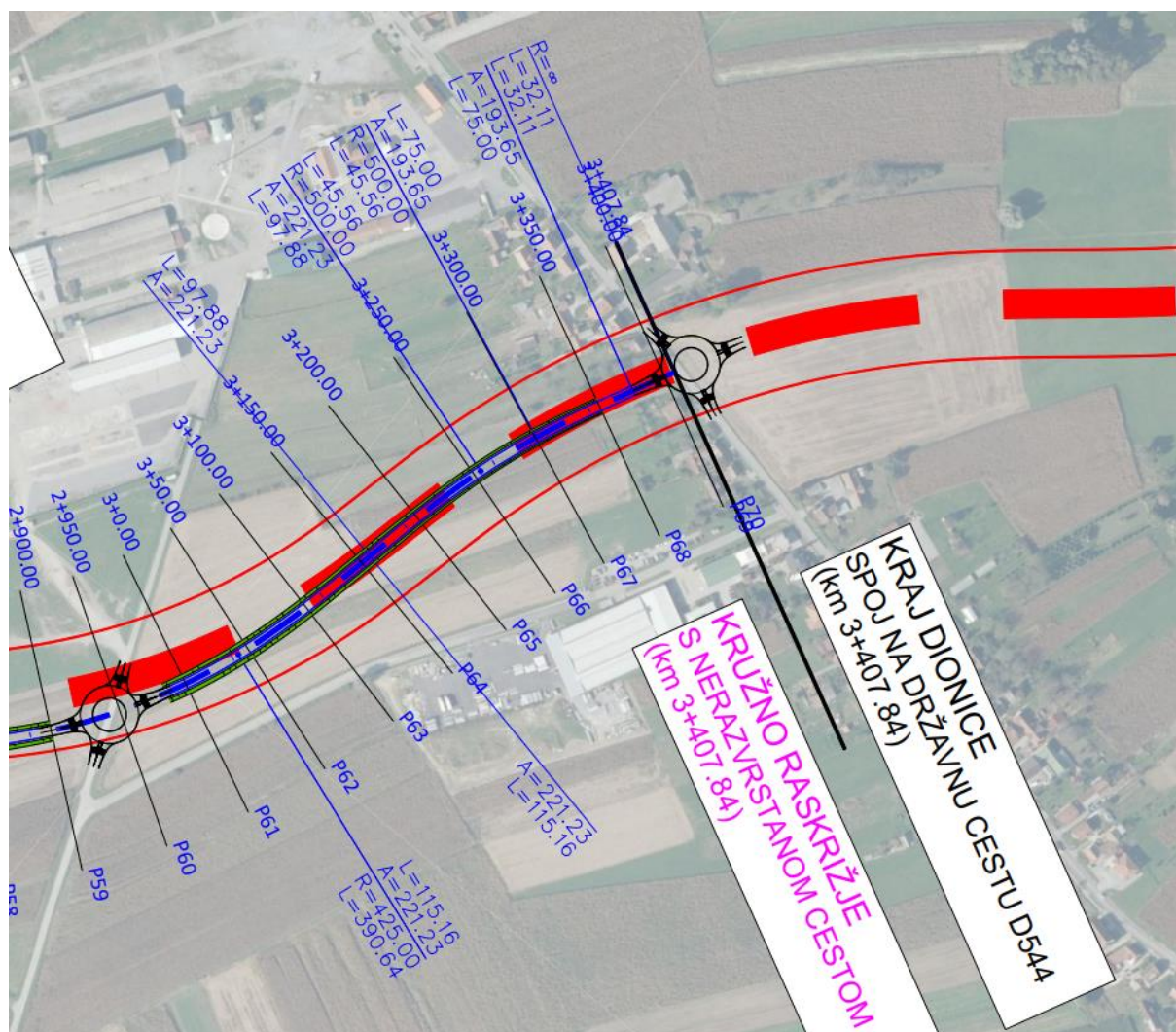
Grafički prikaz B-3: Spoj s državnom cestom DC544 – Varijanta 2 (odabrana varijanta)
