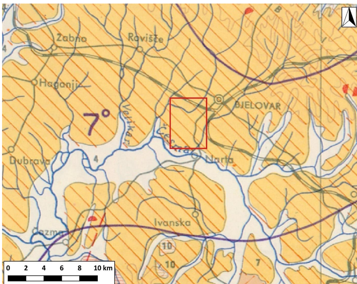
Grafički prikaz C-19: Isječak inženjersko – geološke karte
