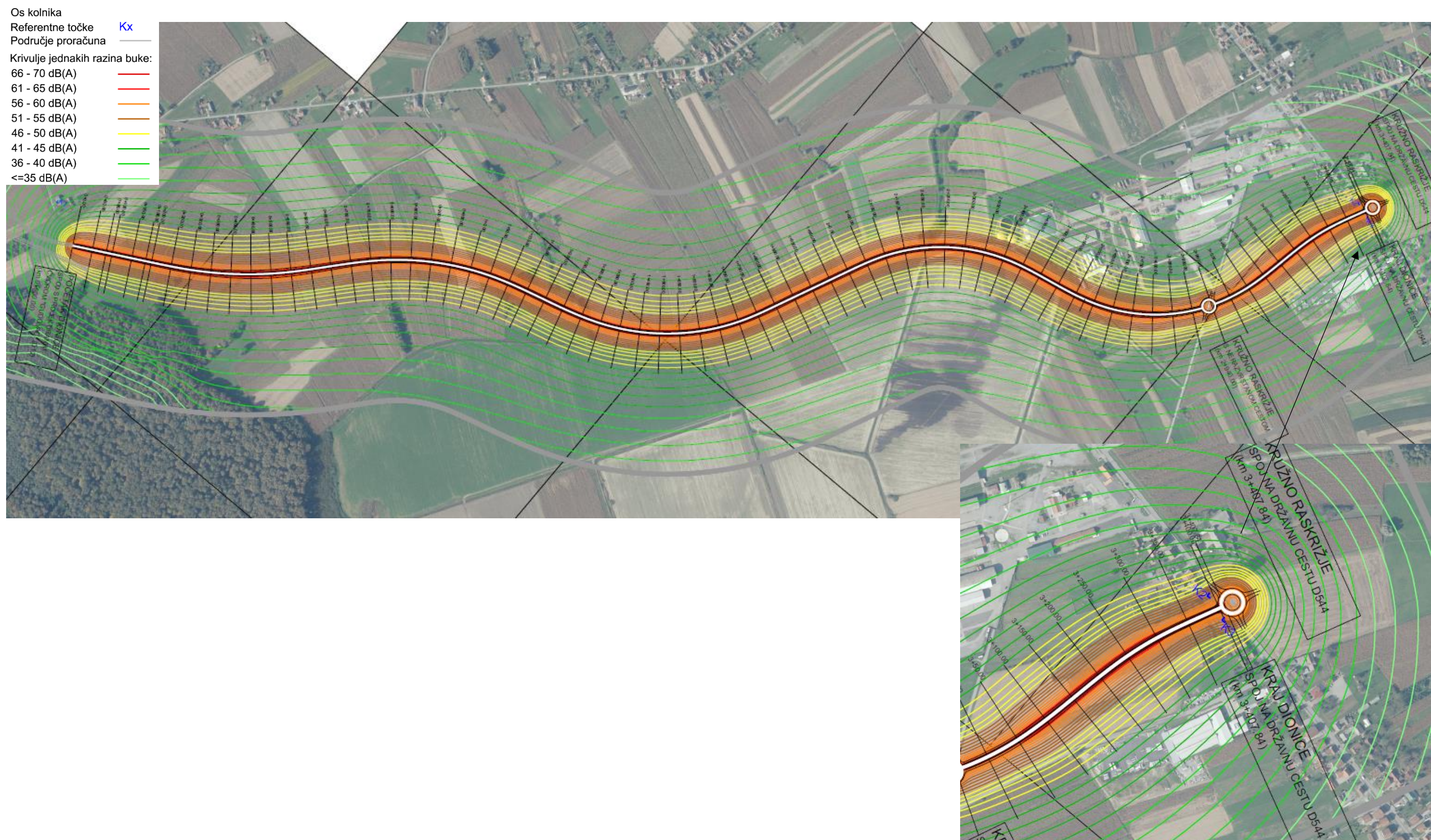
Grafički prikaz D-6: Prikaz širenja buke u okoliš – razdoblje noć – situacija bez zaštite od buke
