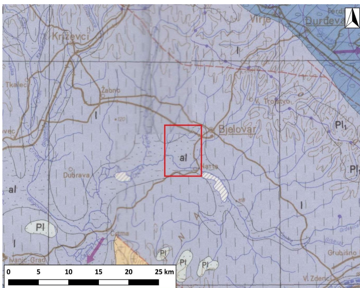
Grafički prikaz C-20: Hidrogeološka karta šireg promatranog područja
