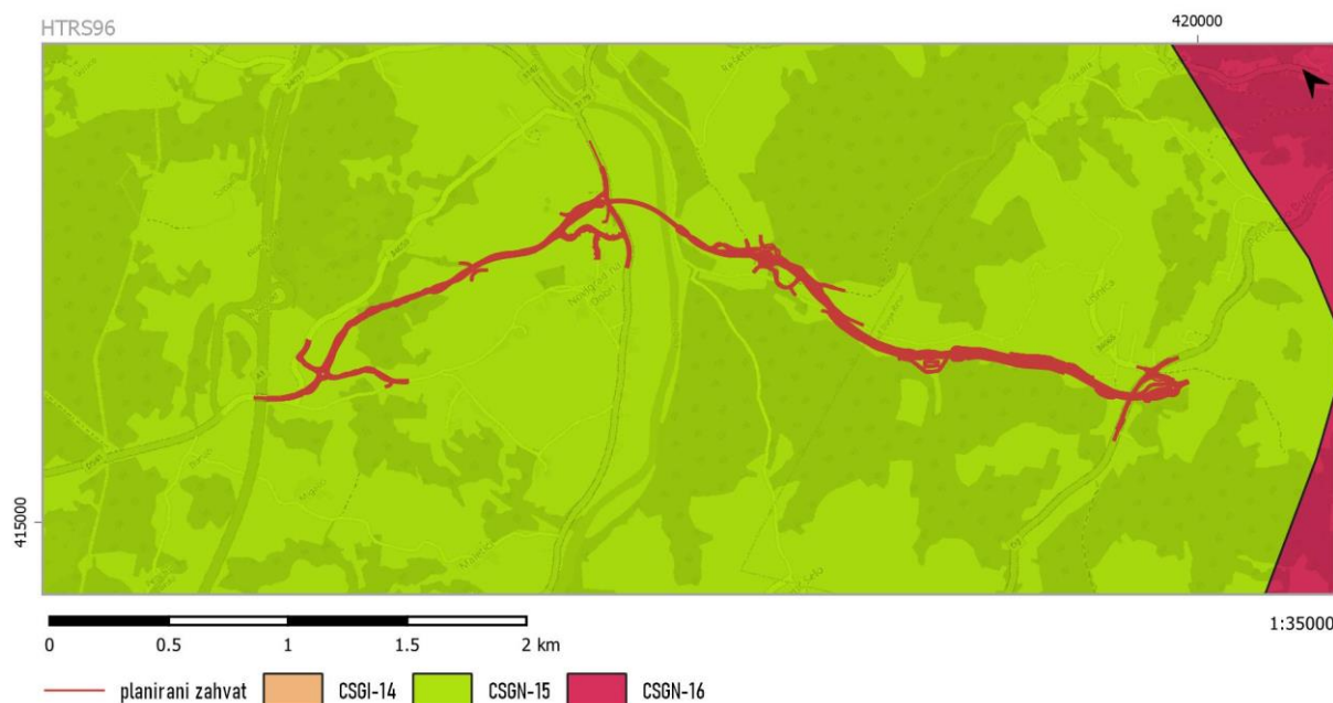
Sl. 3.5-5. Pregledna karta grupiranih vodnih tijela podzemnih voda s označenom lokacijom zahvata (izvor: Plan upravljanja upravljanja vodnim područjima do 2027.)
