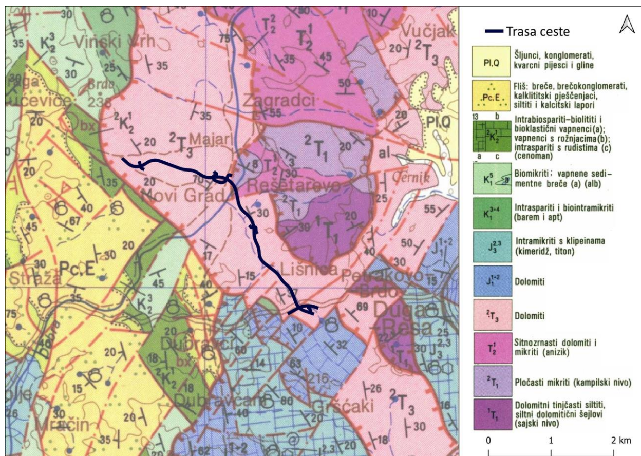
Sl. 3.4-1. Geološka karta šireg područja lokacije zahvata.
