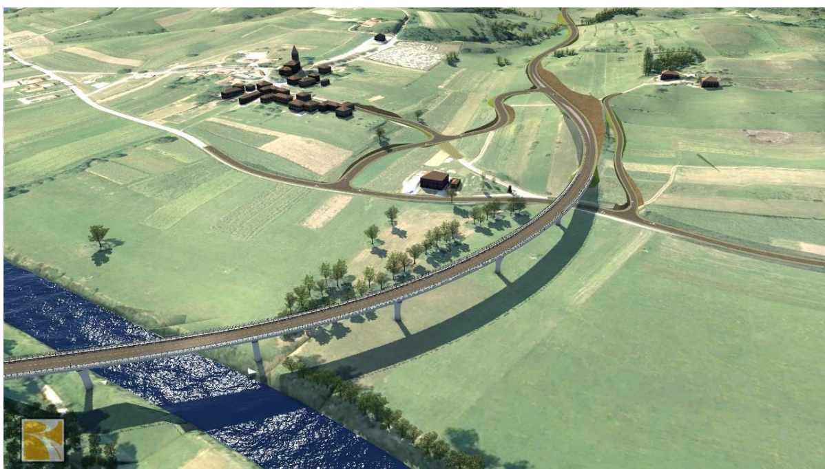
Sl. 1.6-4. Izvadak iz 3D modela: Prikaz mosta viša niveleta (gore) i niža niveleta (dolje)
