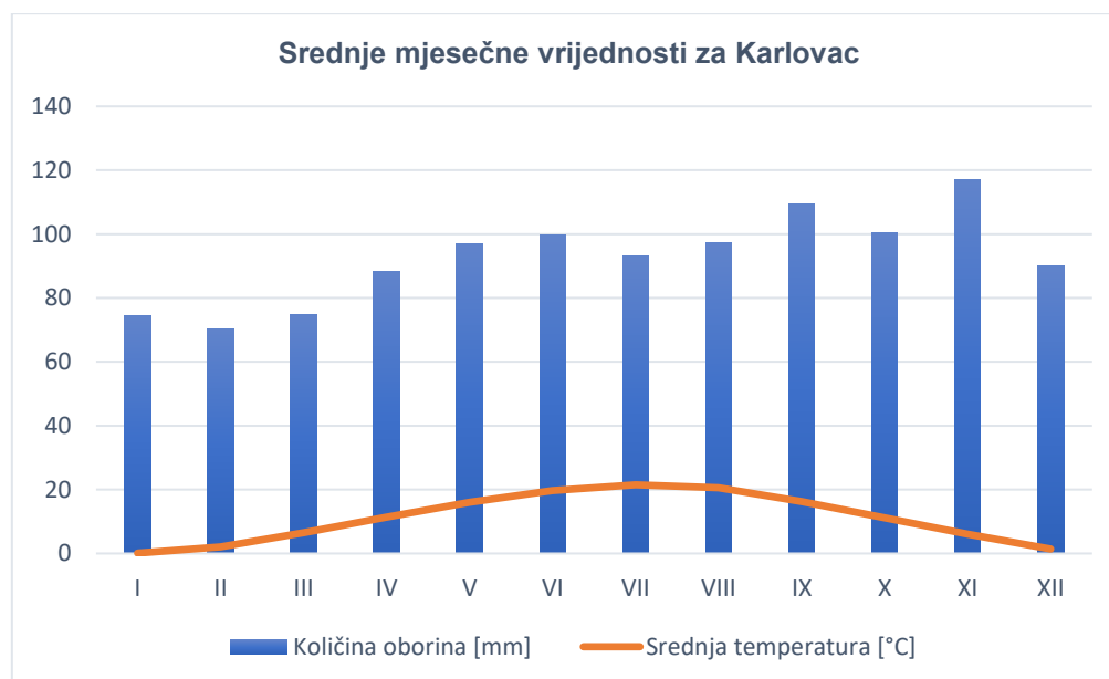
Sl. 3.2-3. Godišnji hod temperature zraka i količine oborine na meteorološkoj postaji Karlovac u razdoblju 1949. – 2019. (Izvor: DHMZ, https://meteo.hr/klima.php?section=klima_podaci&param=k1&Grad=karlovac , obrada: EKONERG d.o.o.)
