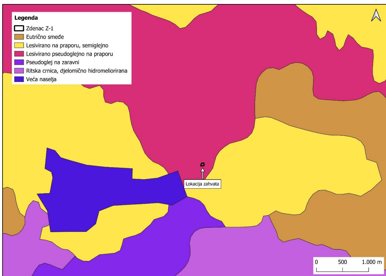
Slika 6. Pedološka obilježja lokacije zahvata (Izvor: envi.azo.hr)
