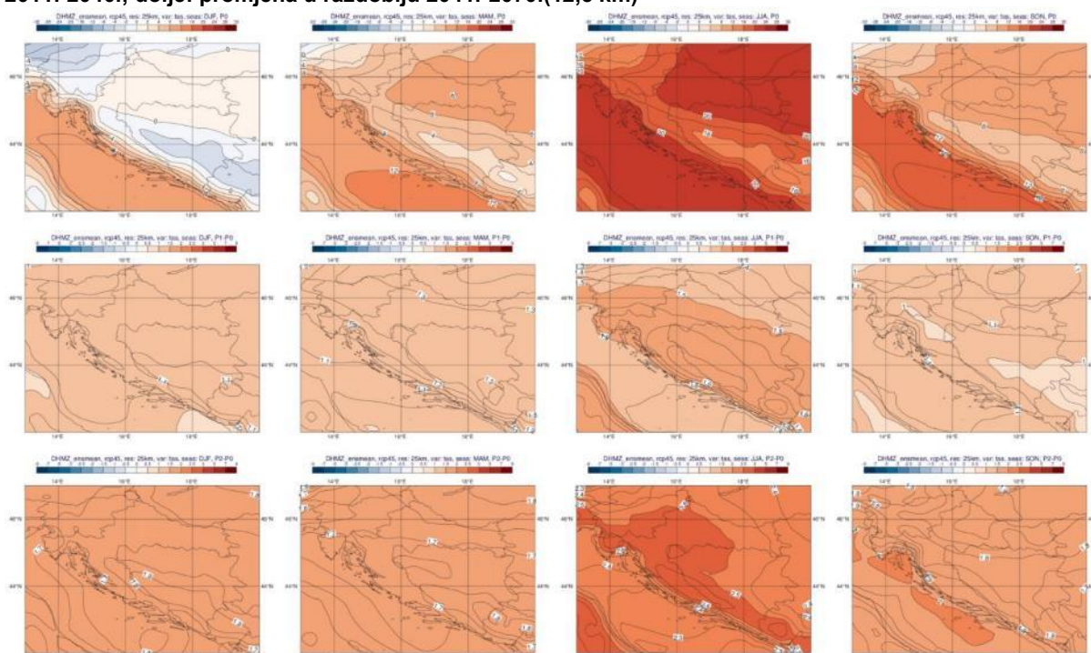
Slika 32. Temperatura zraka (°C) u srednjaku ansambla iz četiri integracije RegCM modelom. Od lijeva na desno: zima, proljeće, ljeto i jesen. Gore: referentno razdoblje 1971.-2000.; sredina: promjena u razdoblju 2011.-2040.; dolje: promjena u razdoblju 2041.-2070.(12,5 km)
