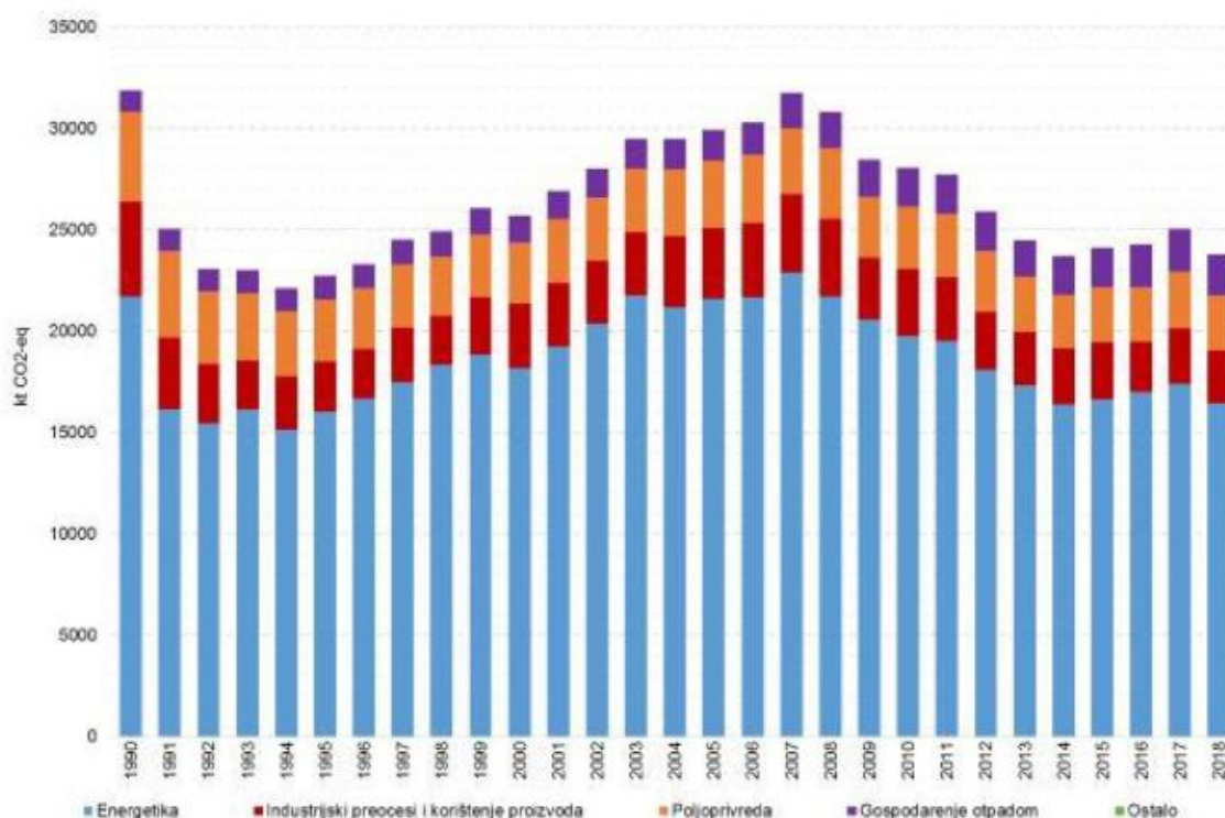
Slika 44. Trend stakleničkih plinova u Republici Hrvatskoj
