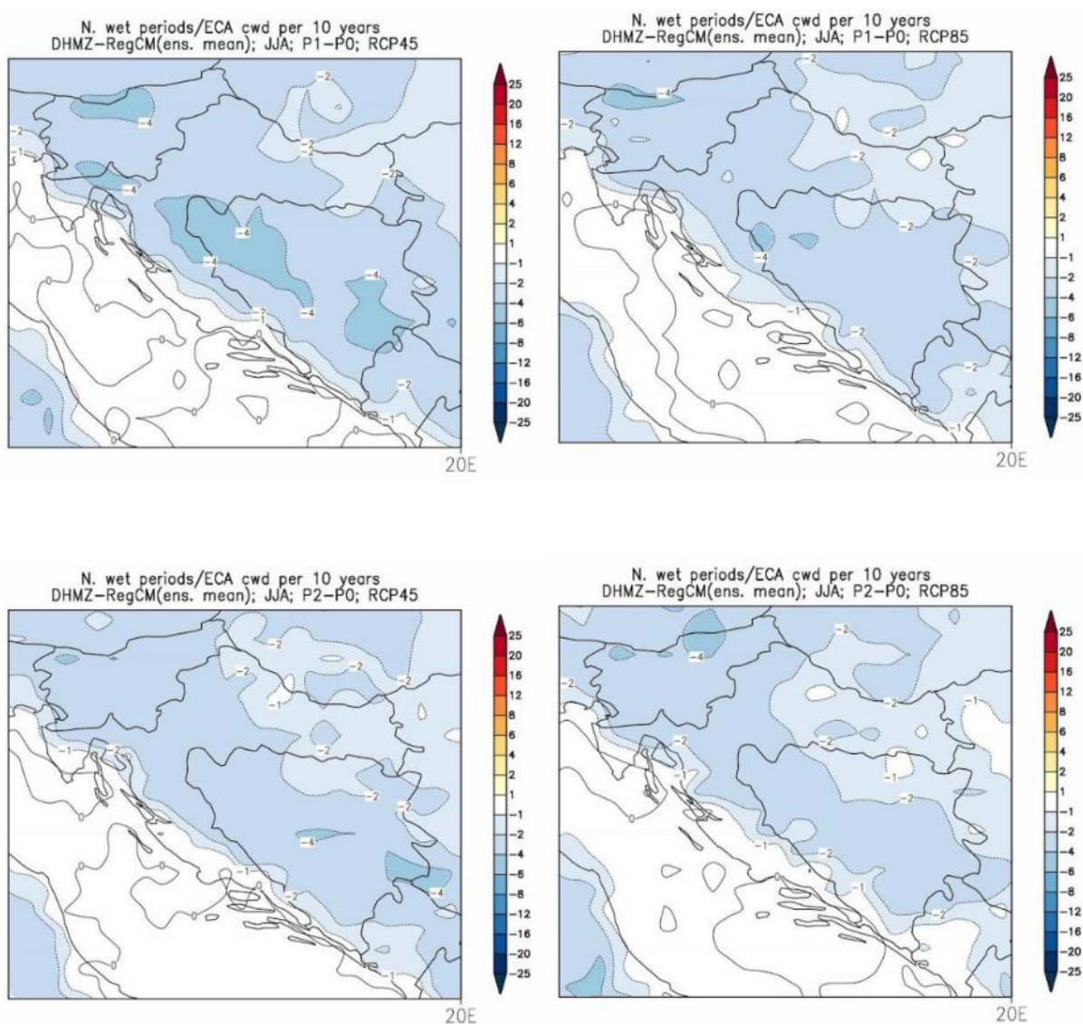
Slika 40. Promjene srednjeg godišnjeg broja kišnih razdoblja u odnosu na referentno razdoblje P0 u srednjaku ansambla iz četiri integracije RegCM modelom. Lijevo scenarij RCP4.5., desno scenarij RCP8.5. Prvi red promjene u razdoblju P1, drugi red promjene u razdoblju P2. Mjerna jedinica broj događaja u 10 godina. Sezona ljeto.(12,5 km)
