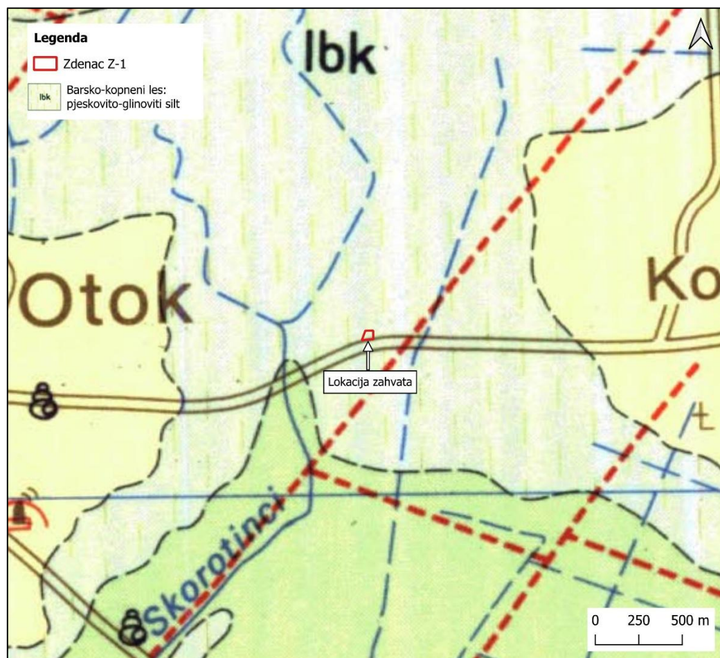
Slika 9. Geološka obilježja lokacije zahvata (Izvor: Hrvatski geološki institut)
