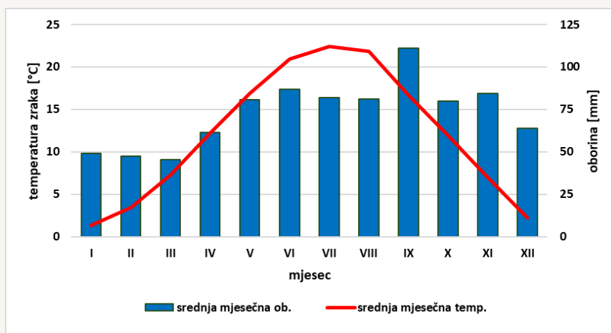
Slika 2.2.1.1. Prikaz srednjih mjesečnih količina oborina, te prosječnih temperatura za područje planiranog zahvata meteorološke postaje Zagreb-Maksimir za razdoblje od 1995. – 2022. godine.
