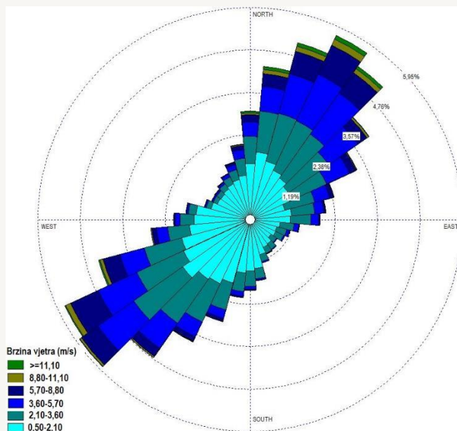
Slika 2.2.1.2. Prikaz godišnje ruže vjetrova za područje planiranog zahvata u razdoblju od 1985. godine do srpnja 2020. godine (Izvor: Meteoblue)
