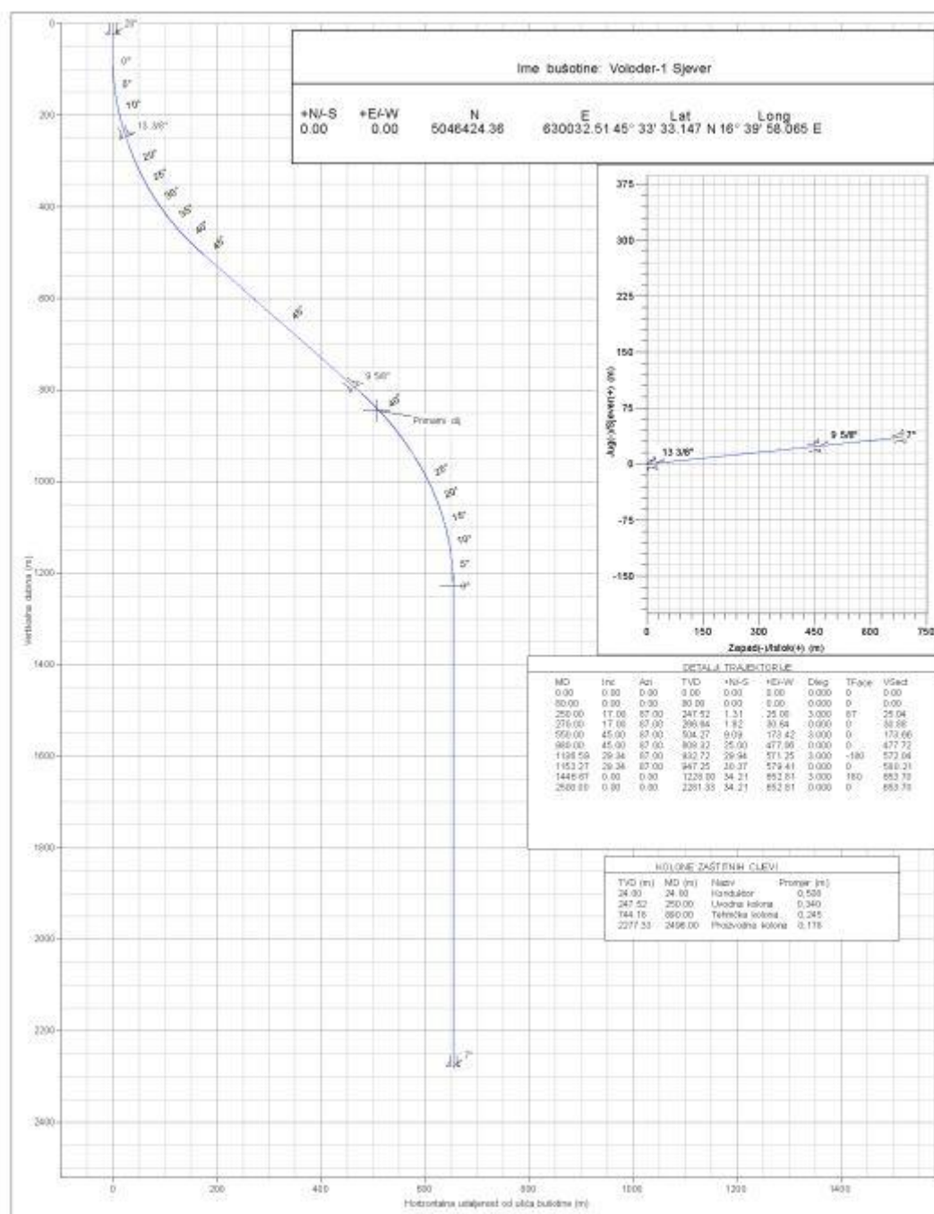
Grafički prikaz 3-7: Trajektorija bušotine Voloder-1 Sjever (Vo-1S)
