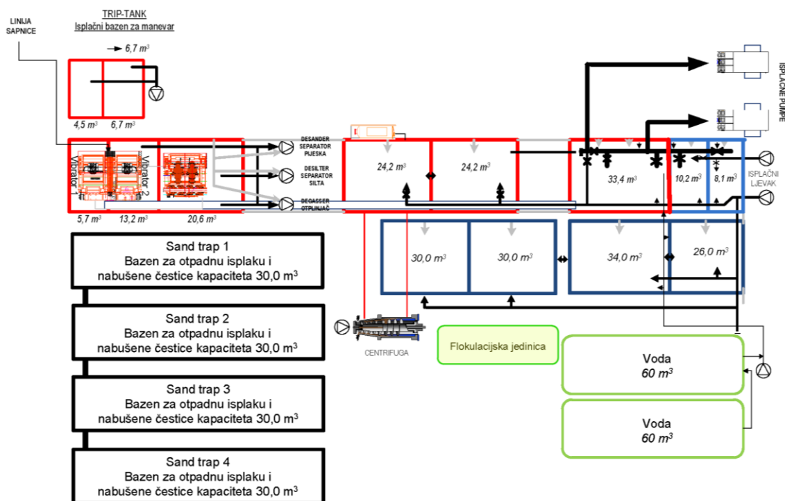
Grafički prikaz 3-6: Shematски prikaz isplačnog sustava bušačeg postrojenja
