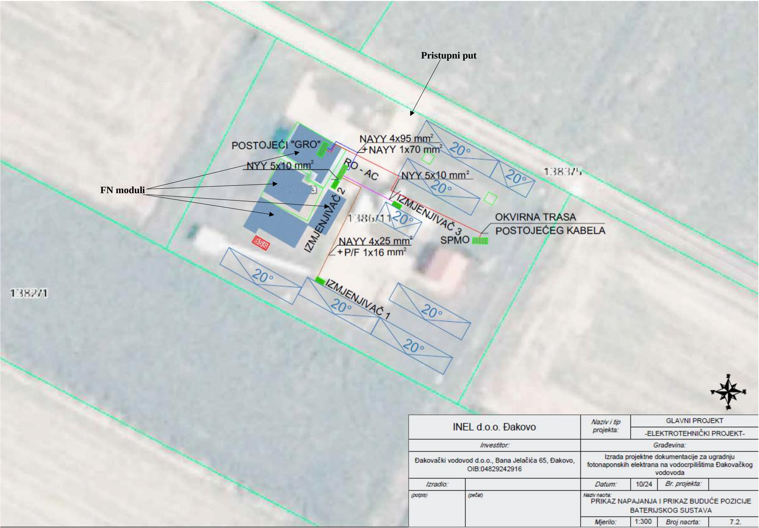
Slika 12. Prikaz napajanja i prikaz buduće pozicije baterijskog sustava (Izvor: IDEJNO RJEŠENJE)
