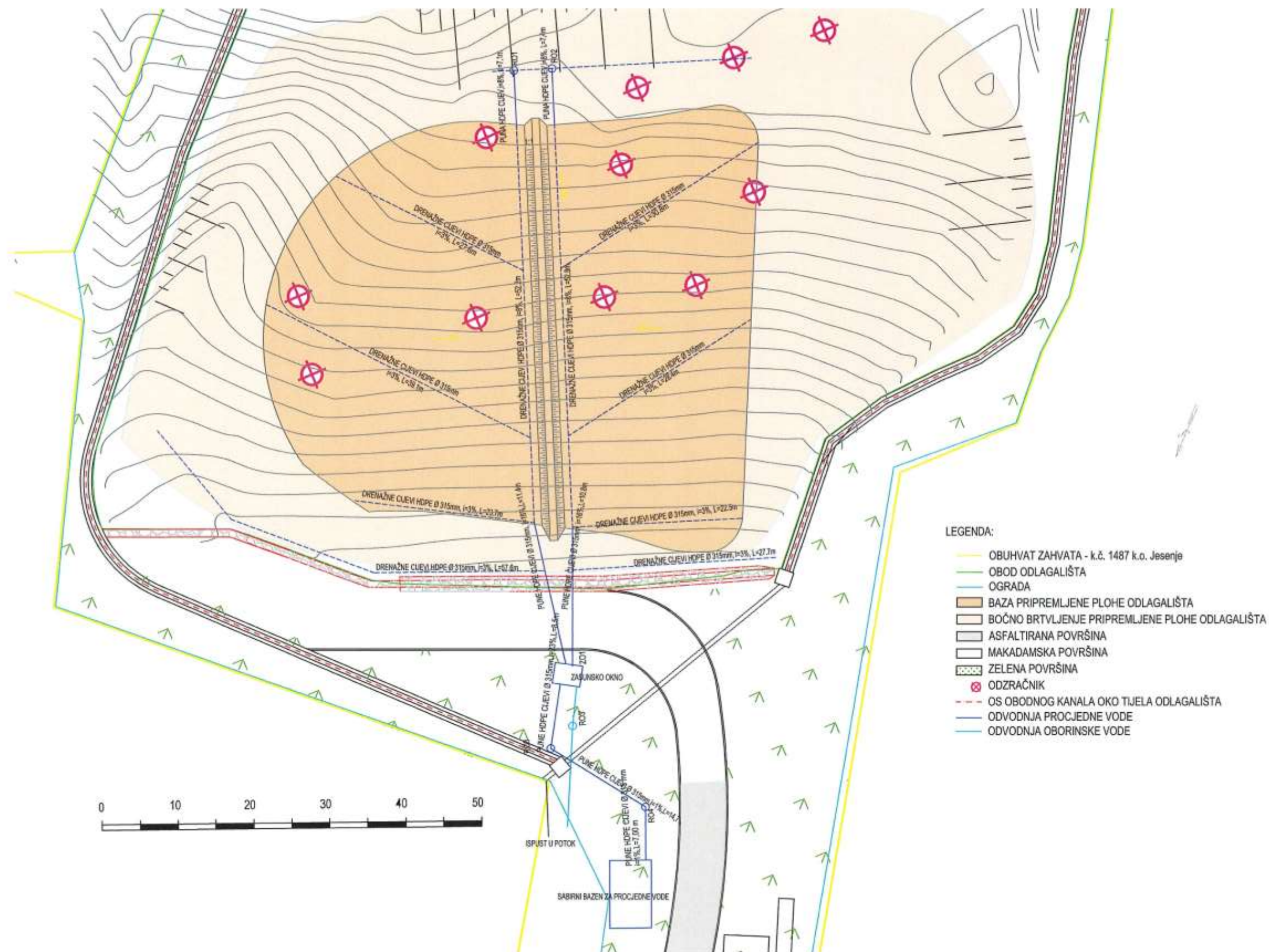
Slika 1.1/2 – Situacija odvodnje procjedne vode s postojeće novoizgrađene (proširene) plohe odlagališta
