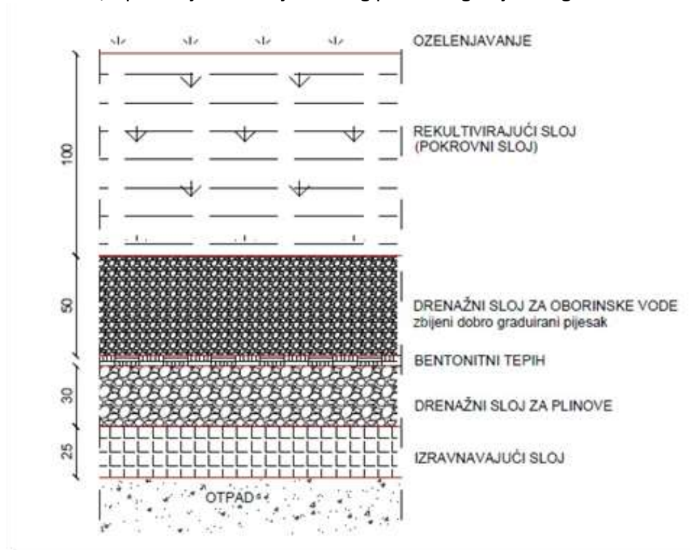
Slika 1.2/2. – Detalj završnog pokrovnog sloja odlagališta
