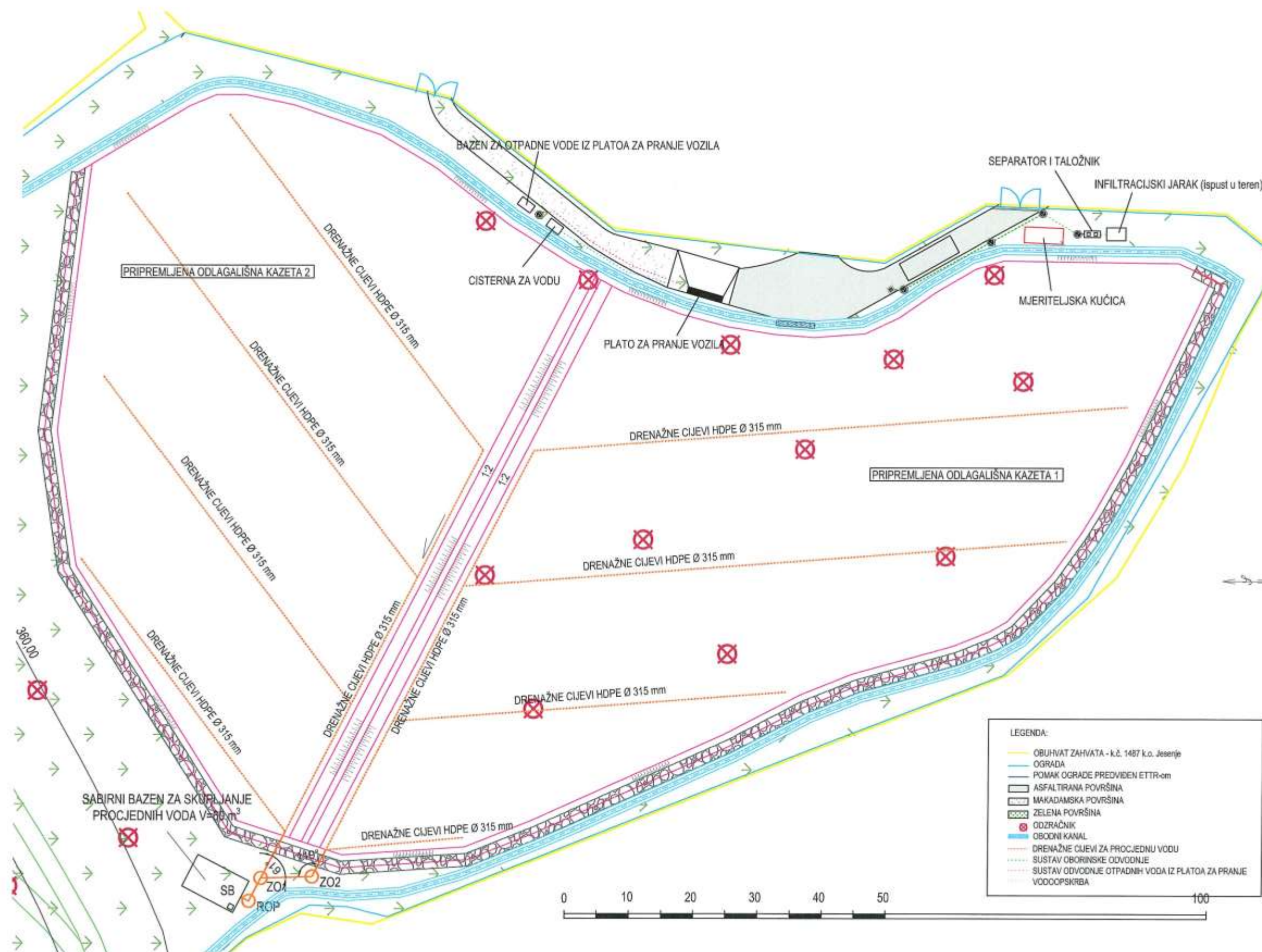
Slika 1.2/5– Situacija odvodnje otpadnih voda s nove ulazno-izlazne zone i procjedne vode s nove pripremljene plohe odlagališta
