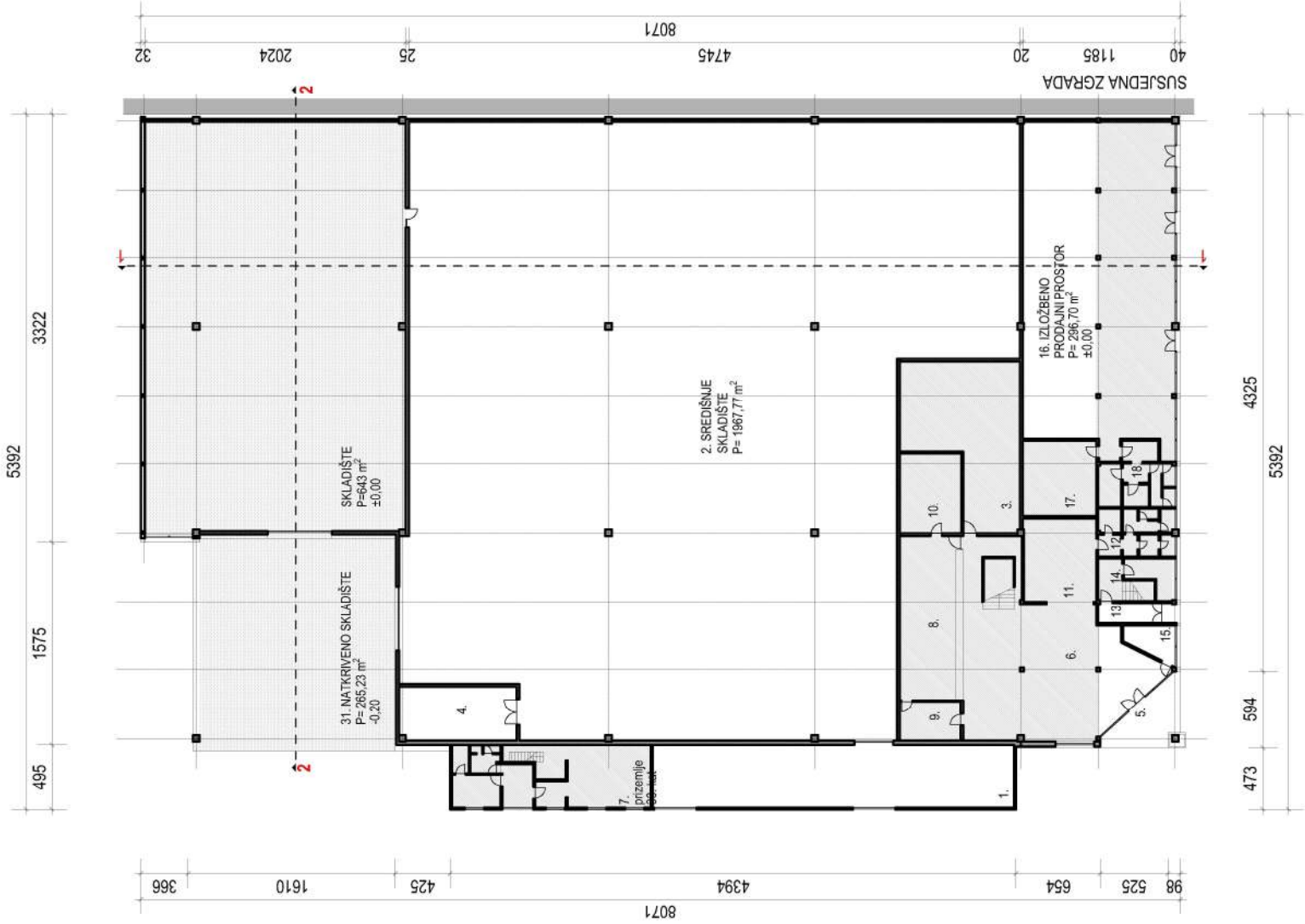
TLOCRT PRIZEMLJA
