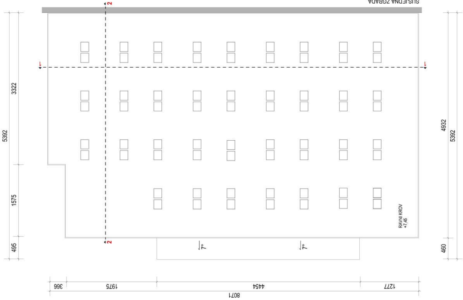
TLOCRT KROVA
