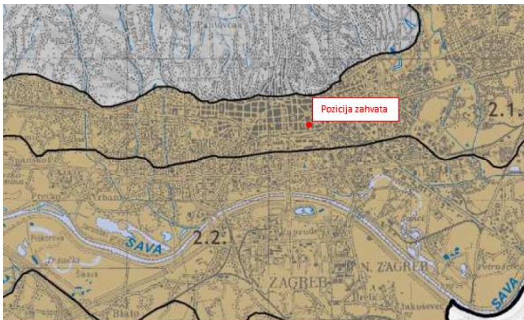
Slika 2.21. Isječak iz karte Opća tipologija krajobraza. Izvor: Studija zaštite karaktera krajobraza Grada Zagreba, Oikon 2015.
