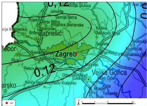
Slika 2.19 Karta za povratno razdoblje za 95 g (Izvor: http://seizkarta.gfz.hr/karta.php )
