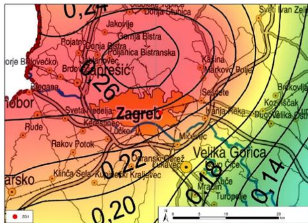
Slika 2.20 Karta za povratno razdoblje za 475 g (Izvor: http://seizkarta.gfz.hr/karta.php )
