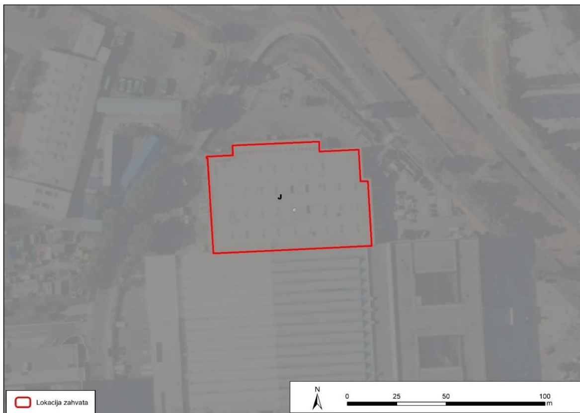
Slika 2.22 Karta prirodnih, poluprirodnih i kopnenih ne-šumskih staništa na djelu obuhvata predloženog zahvata 2016 – pregledna karta (Izvor: www.bioportal.hr )
