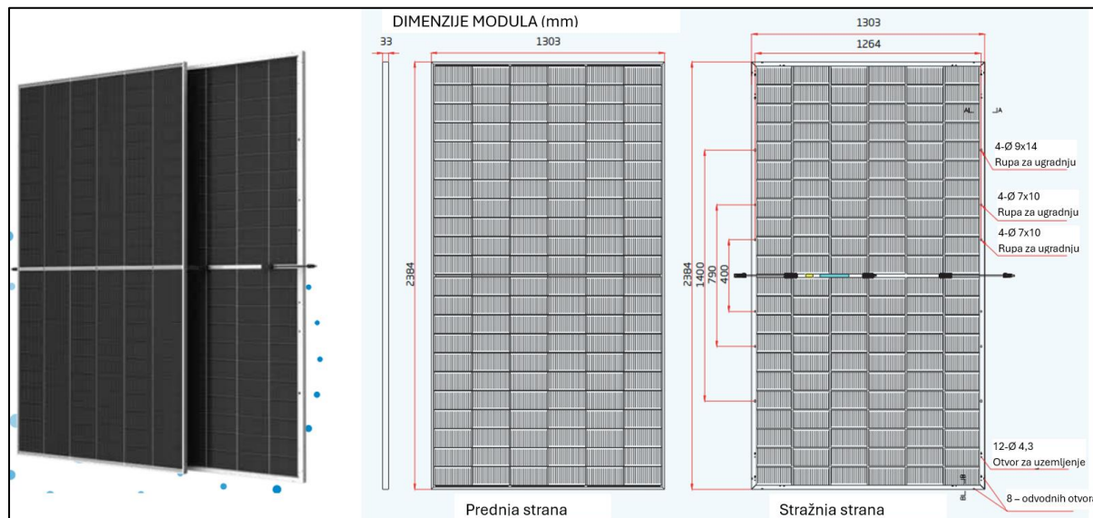
Slika 3. Prikaz fotonaponskog panela
