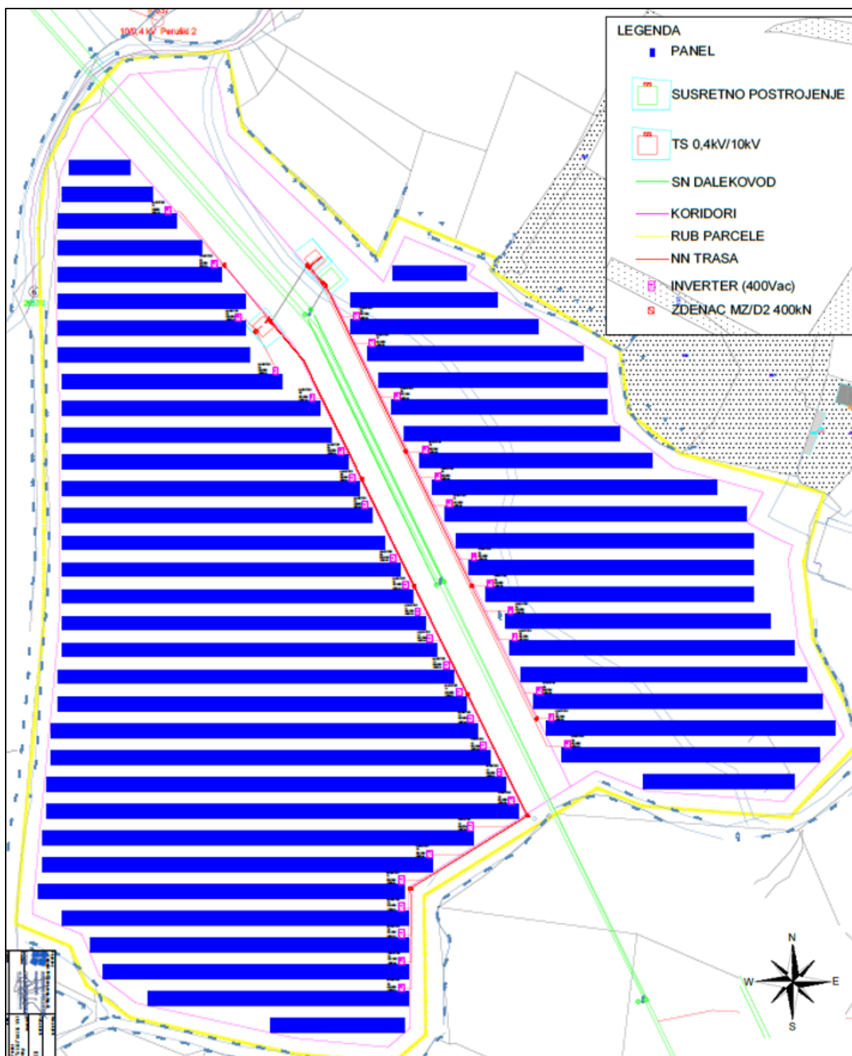
Slika 2. Prikaz dispozicije opreme na lokaciji zahvata
