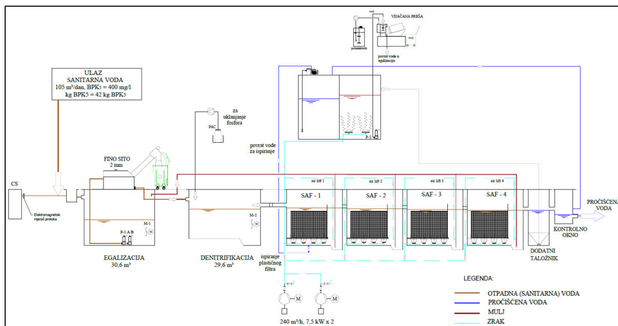
Slika 13. Tehnološka shema UPOV-a Cerovlje (izvor: Idejni projekt)
