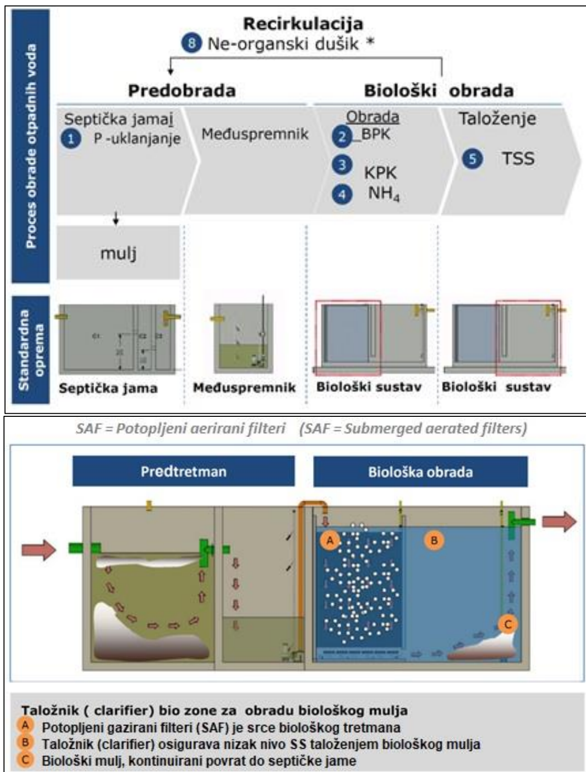
Slika 12. Proces obrade otpadnih voda SAF tehnologijom
