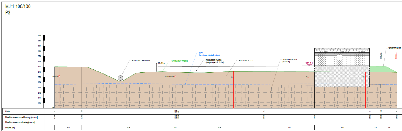
Slika 10. Prikaz presjeka kroz plato UPOV-a Cerovlje, profil 3 (izvor: idejni projekt)
