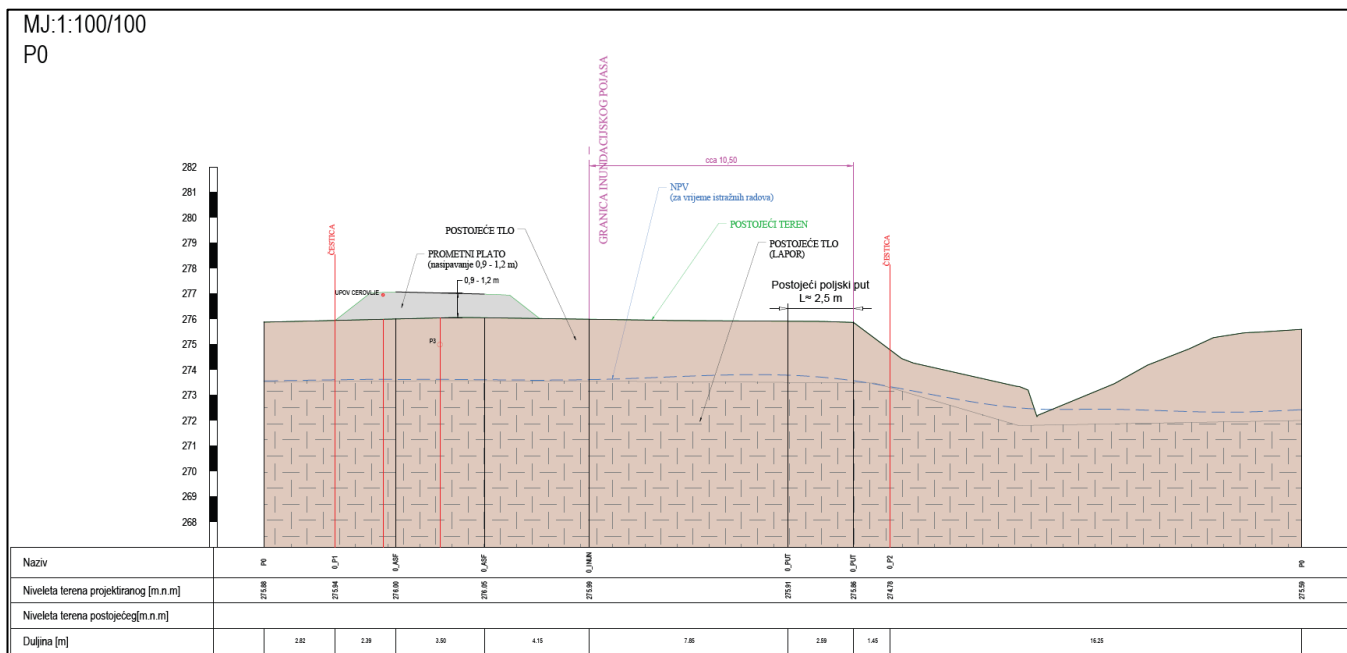
Slika 7. Prikaz presjeka kroz plato UPOV-a Cerovlje, profil 0 (izvor: idejni projekt)
