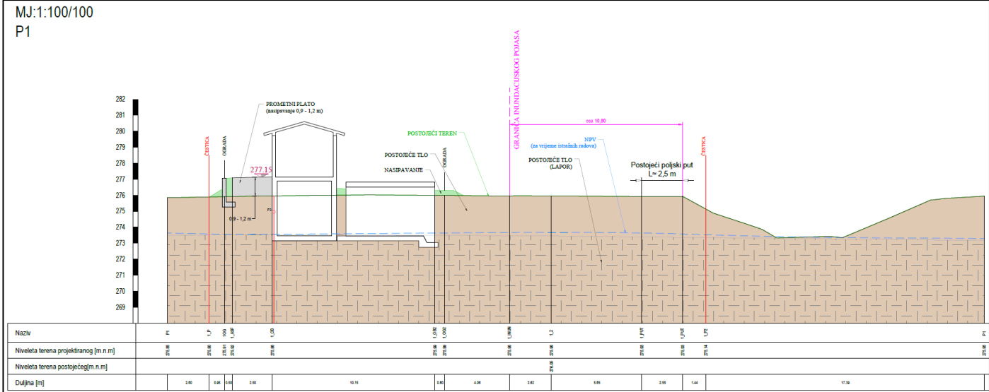
Slika 8. Prikaz presjeka kroz plato UPOV-a Cerovlje, profil 1 (izvor: idejni projekt)
