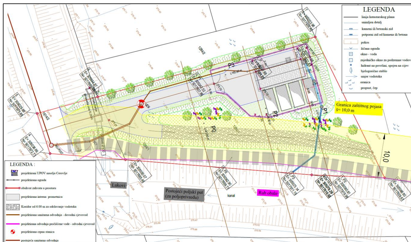
Slika 6. Prikaz situacije UPOV-a Cerovlje (izvor: idejni projekt)
