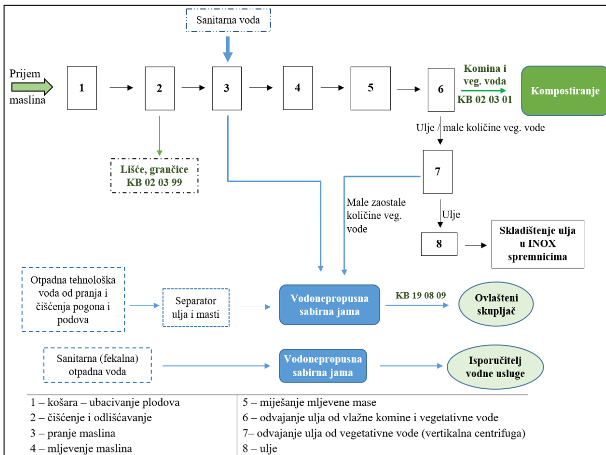
Slika 6. Shema tehnološkog procesa s prikazom emisija u okoliš i nastankom otpadnih tvari
