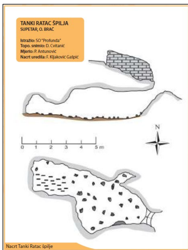
Slika 16 Nacrt Špilje u Tankom Ratcu
