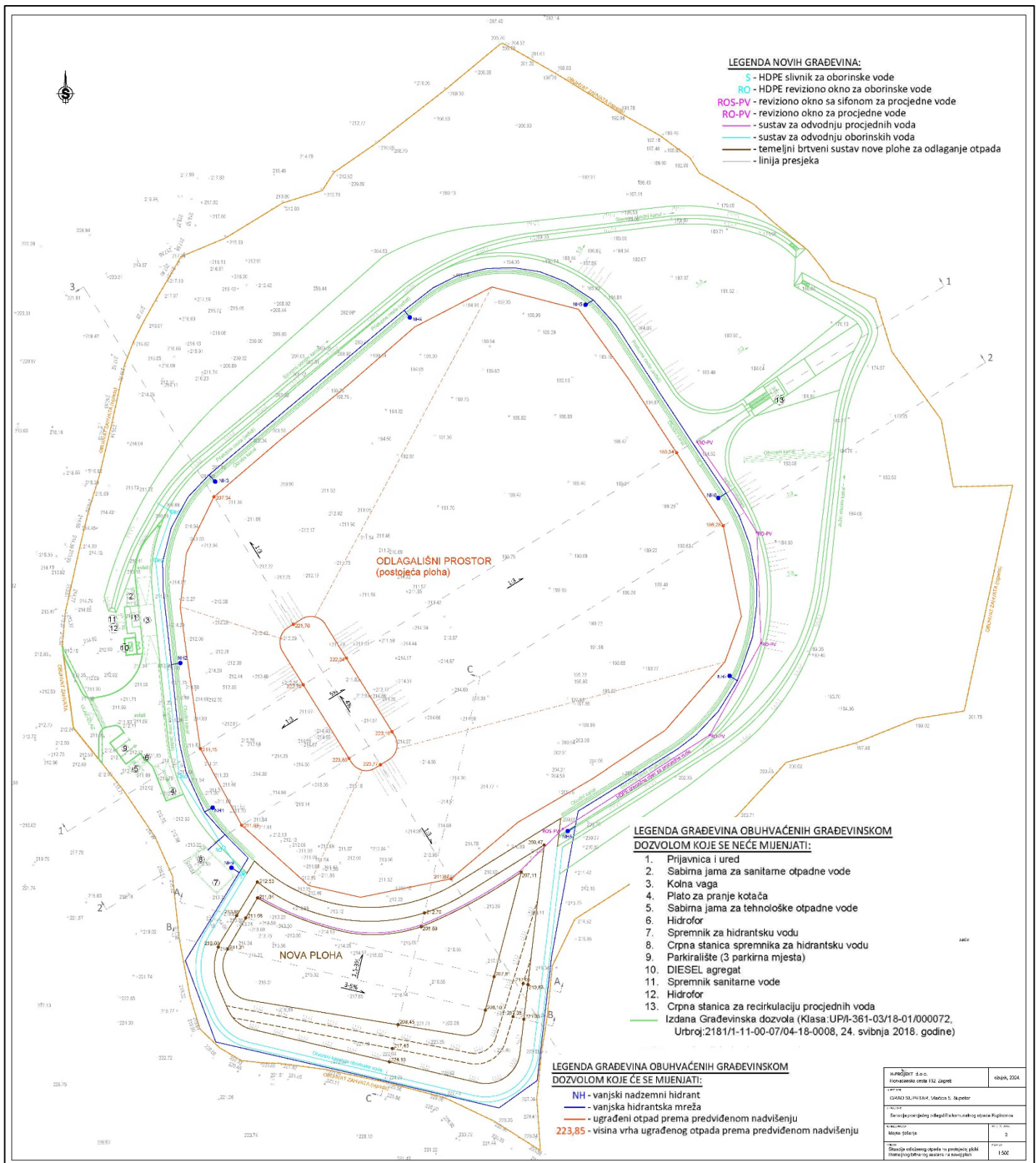
Slika 2 Situacijski prikaz planiranih izmjena EZO 2024.
