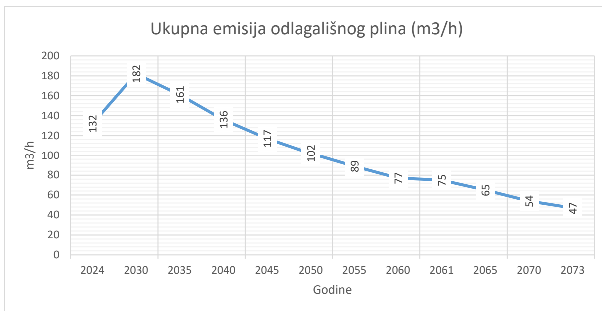
Slika 6 Projekcija količine stvaranja odlagališnog plina (Početak odlaganja u 2024. Predviđeno vrijeme rada 6 godina)
