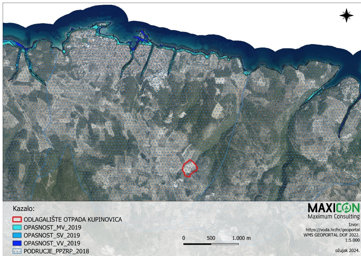
Slika 11 Prikaz lokacije zahvata u odnosu na područja male, srednje i velike učestalosti pojavljivanja poplava
