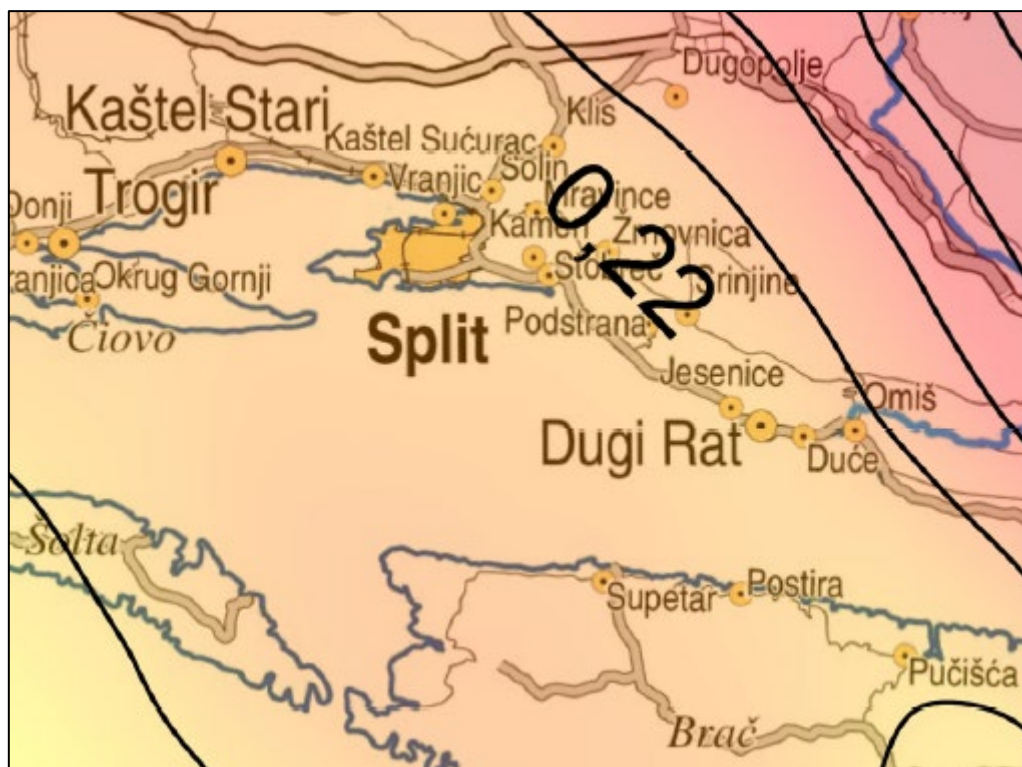
Slika 9 Vršna ubrzanja tla uzrokovana potresima za povratni period za 475 godina (izvor: Karta potresnih područja RH)
