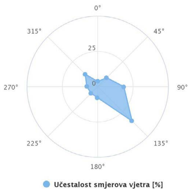
Slika 3.2.9 Učestalost smjerova vjetra
