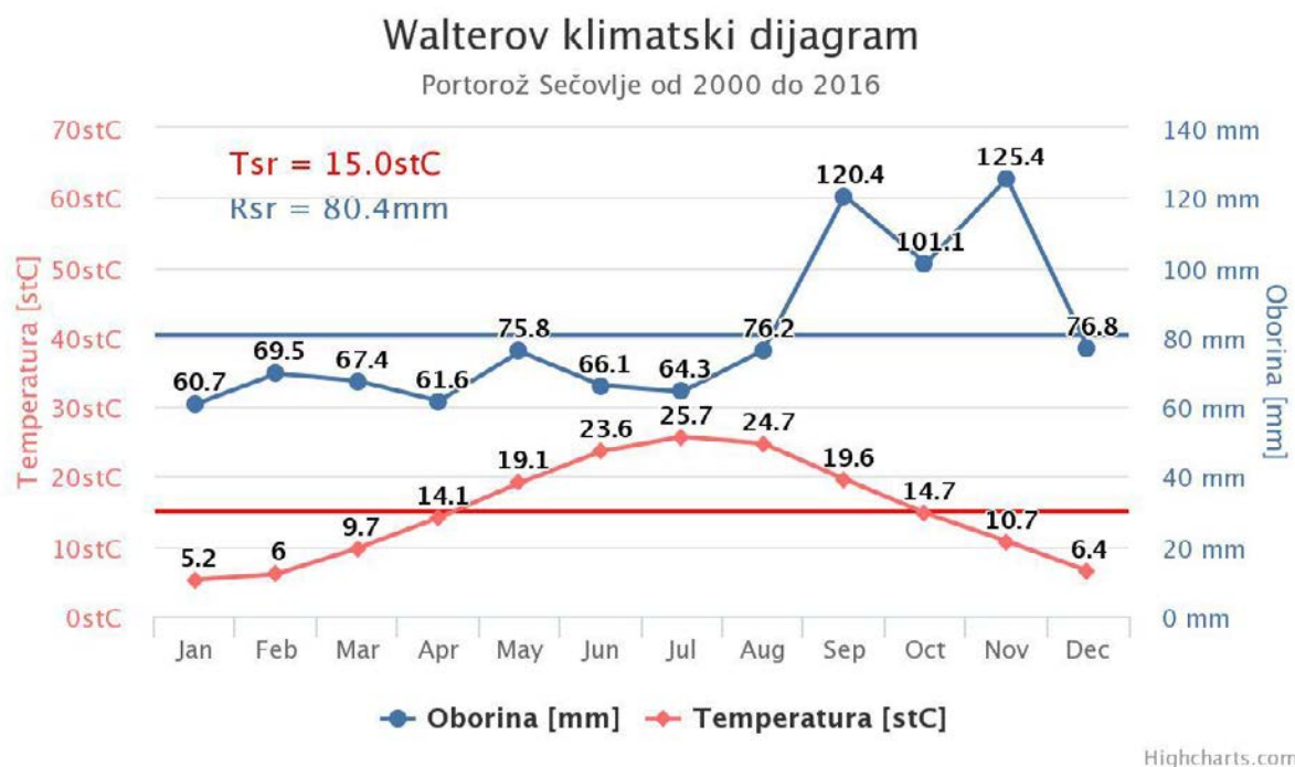
Slika 3.2.8 Walterov klimatski dijagram
