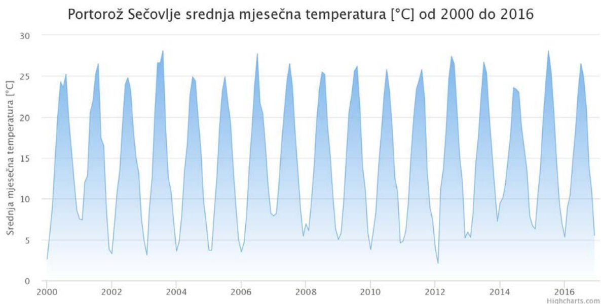
Slika 3.2.2 Srednje mjesečne temperature zraka
