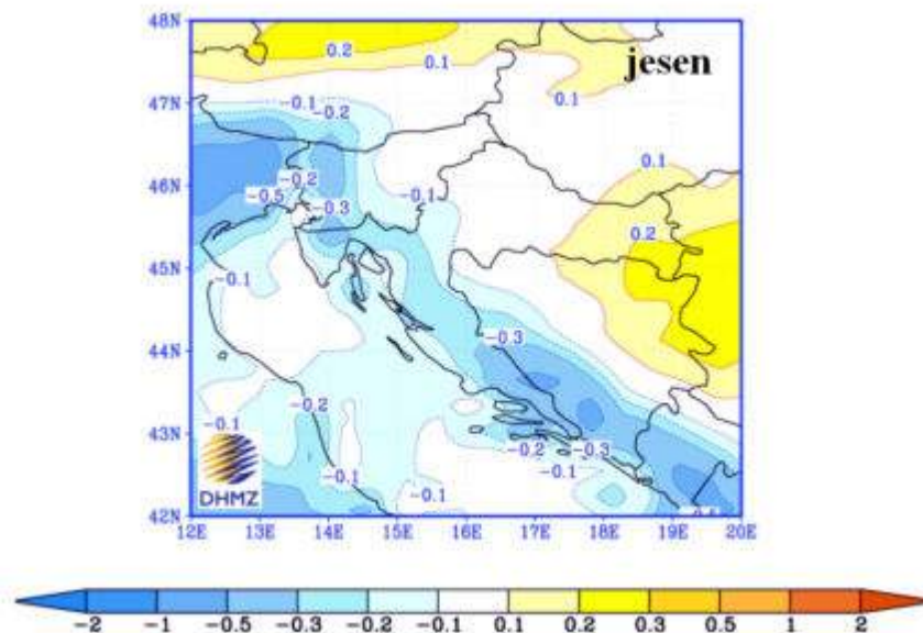
Slika 3.1.8.3: Promjene količine oborine u bližoj budućnosti (prvo razdoblje 2011. - 2040.)
