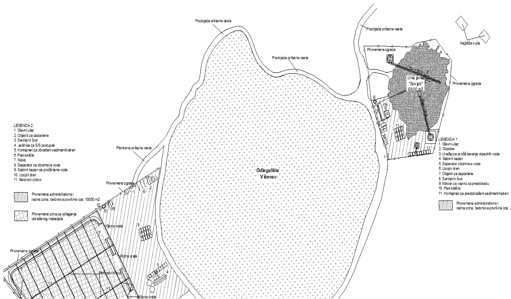
Slika 2.1-2. Situacija Varijante 3 (stabilizacija/solidifikacija mekog katrana)
