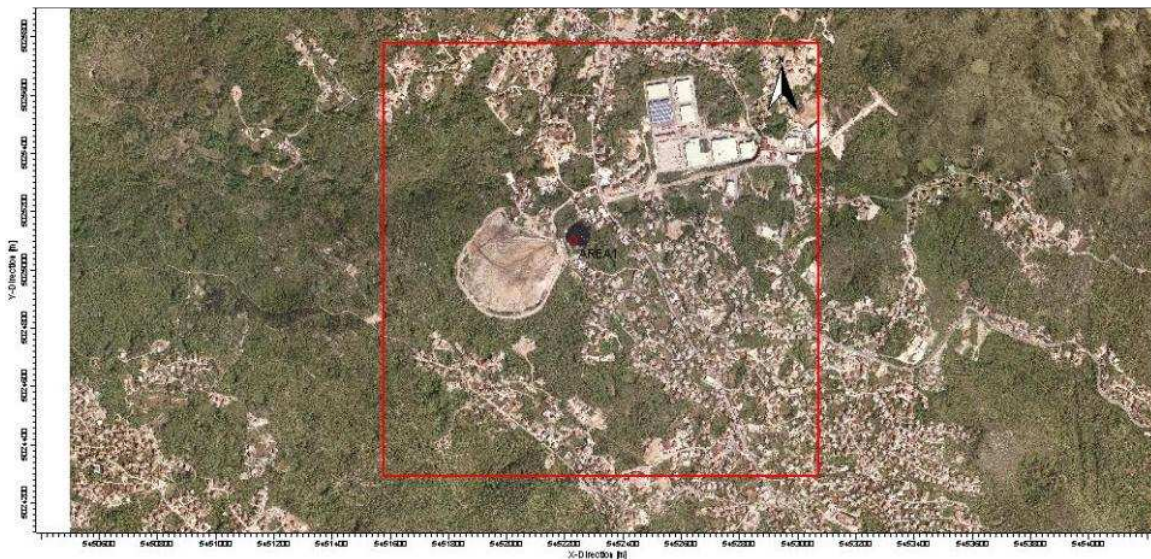
Slika 4.1.-1. Crveni kružić označava položaj izvora u modelu. Domena modela označeno je crvenim pravokutnikom
