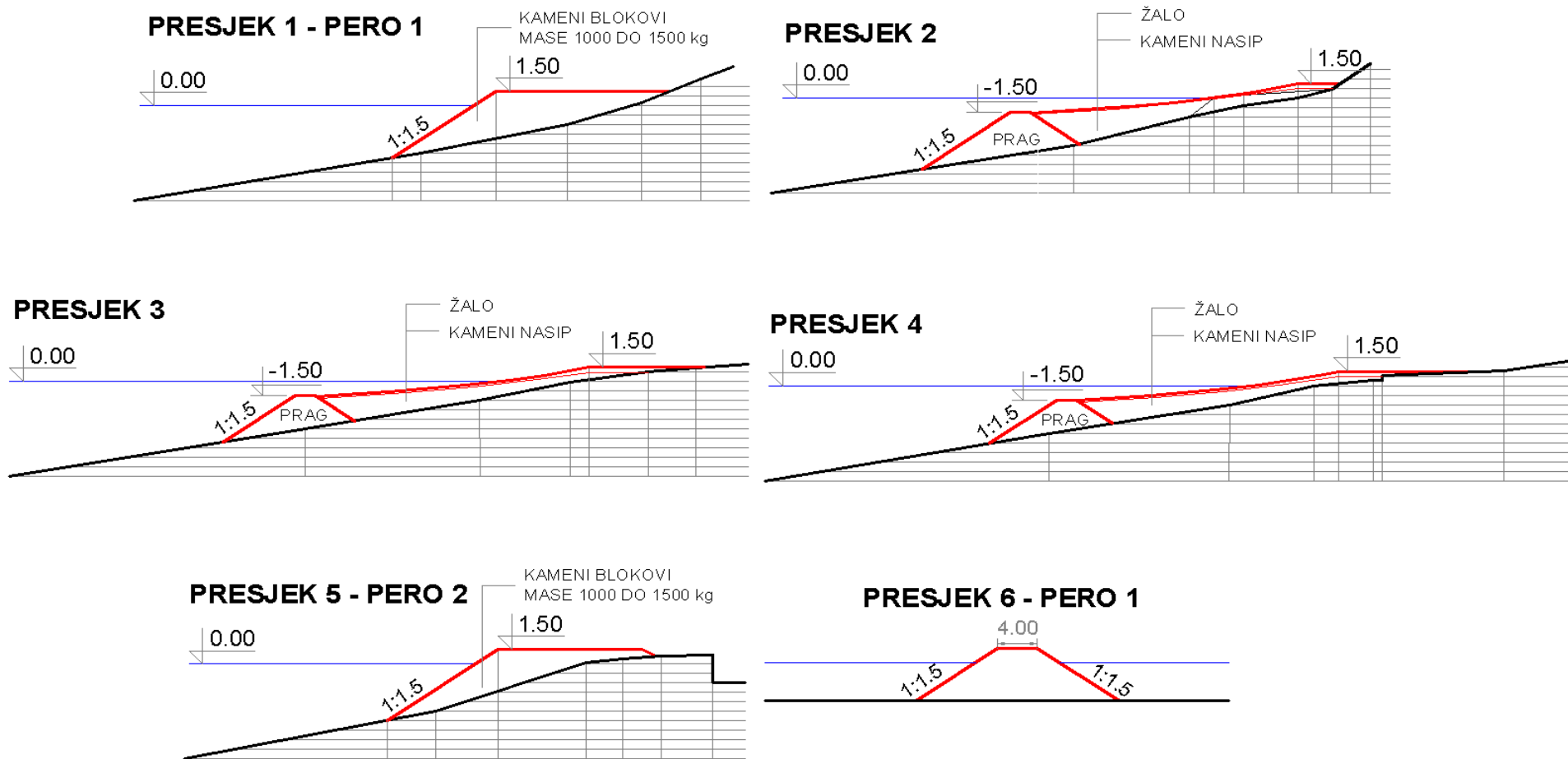
Slika 1.7. Poprečni presjeci pera i lica plaže
