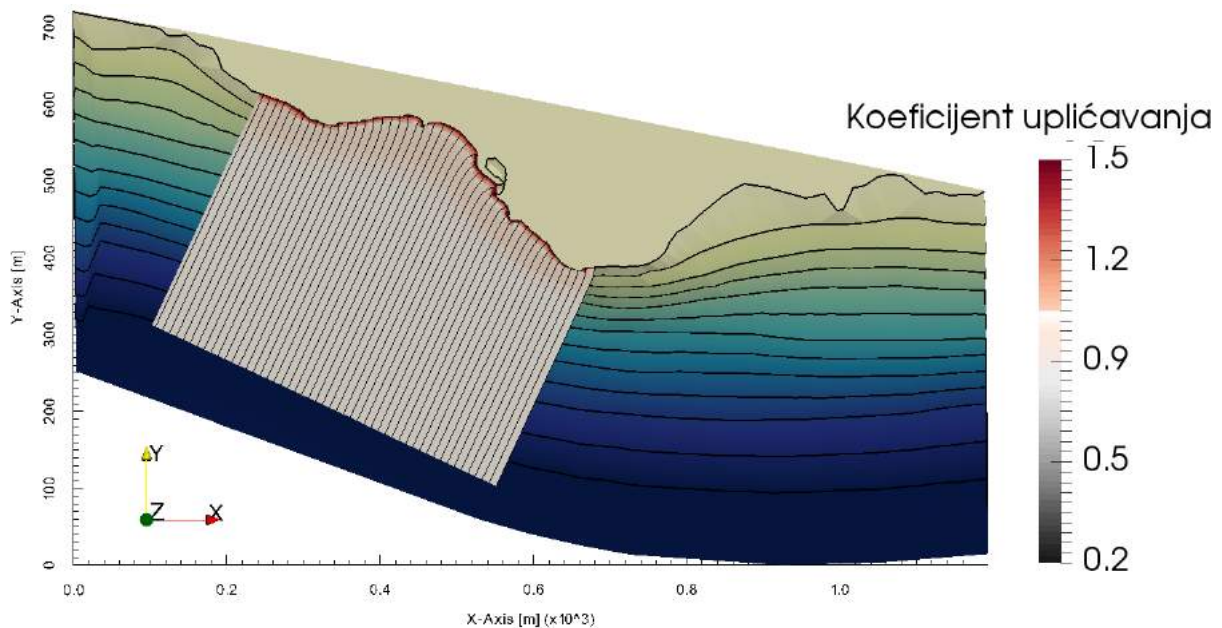
Slika 2.11. Utjecaj uplićavanja vala za Sektor II ( H_s^5=1.73 m, T_0^5=4.88 s)
