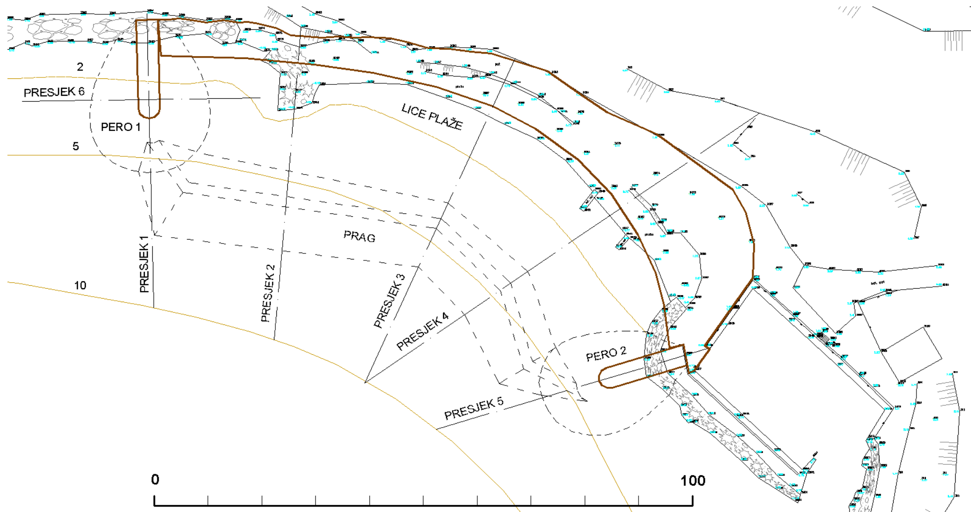
Slika 1.6. Situacija uređenja plaže
