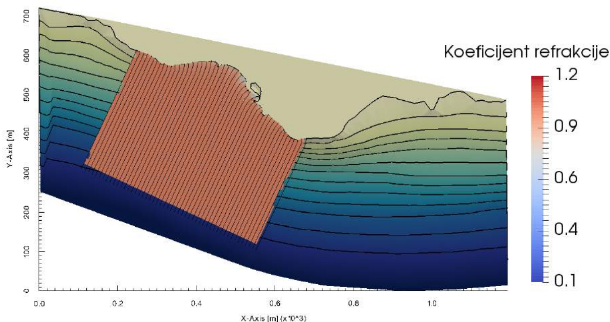
Slika 2.9. Plan refrakcije za Sektor II ( H_s^5=1.73\text{ m} , T_0^5=4.88\text{ s} )
