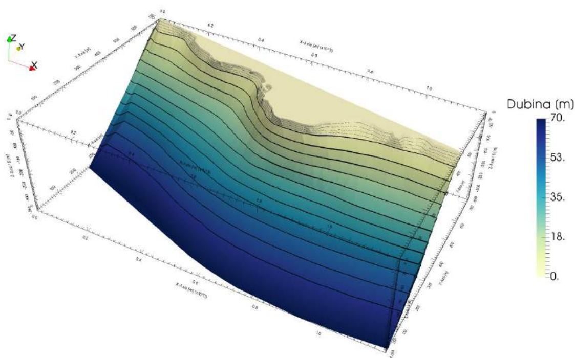
Slika 2.6. 3D prikaz morskog dna za prošireni akvatorij uvale Vojskovo
