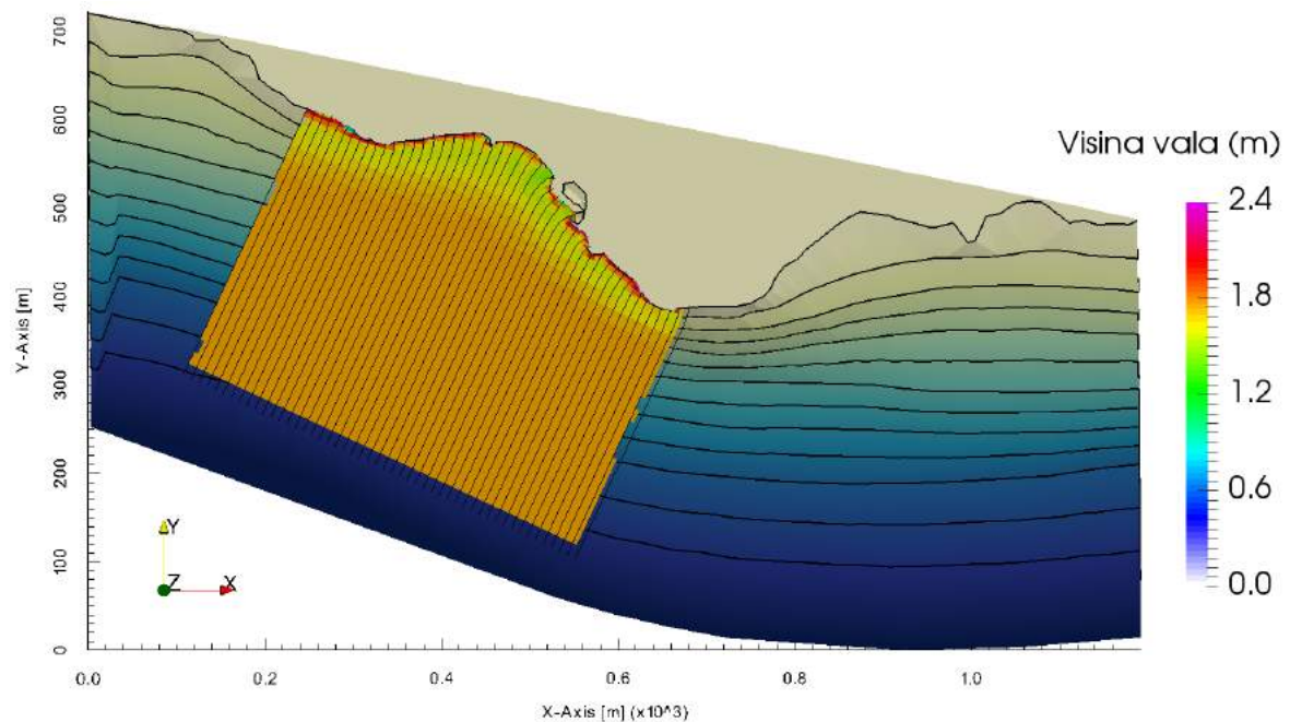
Slika 2.15. Polje značajnih visina vala za Sektor II ( H_s^5=1.73 m, T_0^5=4.88 s)
