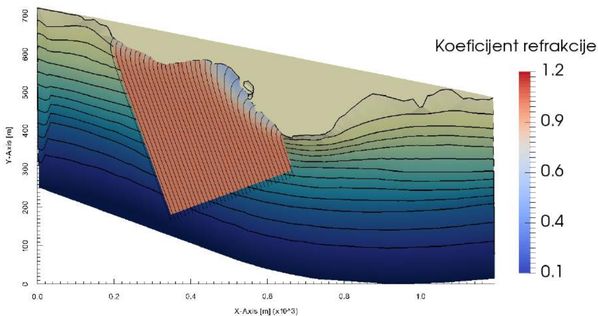
Slika 2.8. Plan refrakcije za Sektor I ( H_s^5=2.12\text{ m} , T_0^5=5.40\text{ s} )
