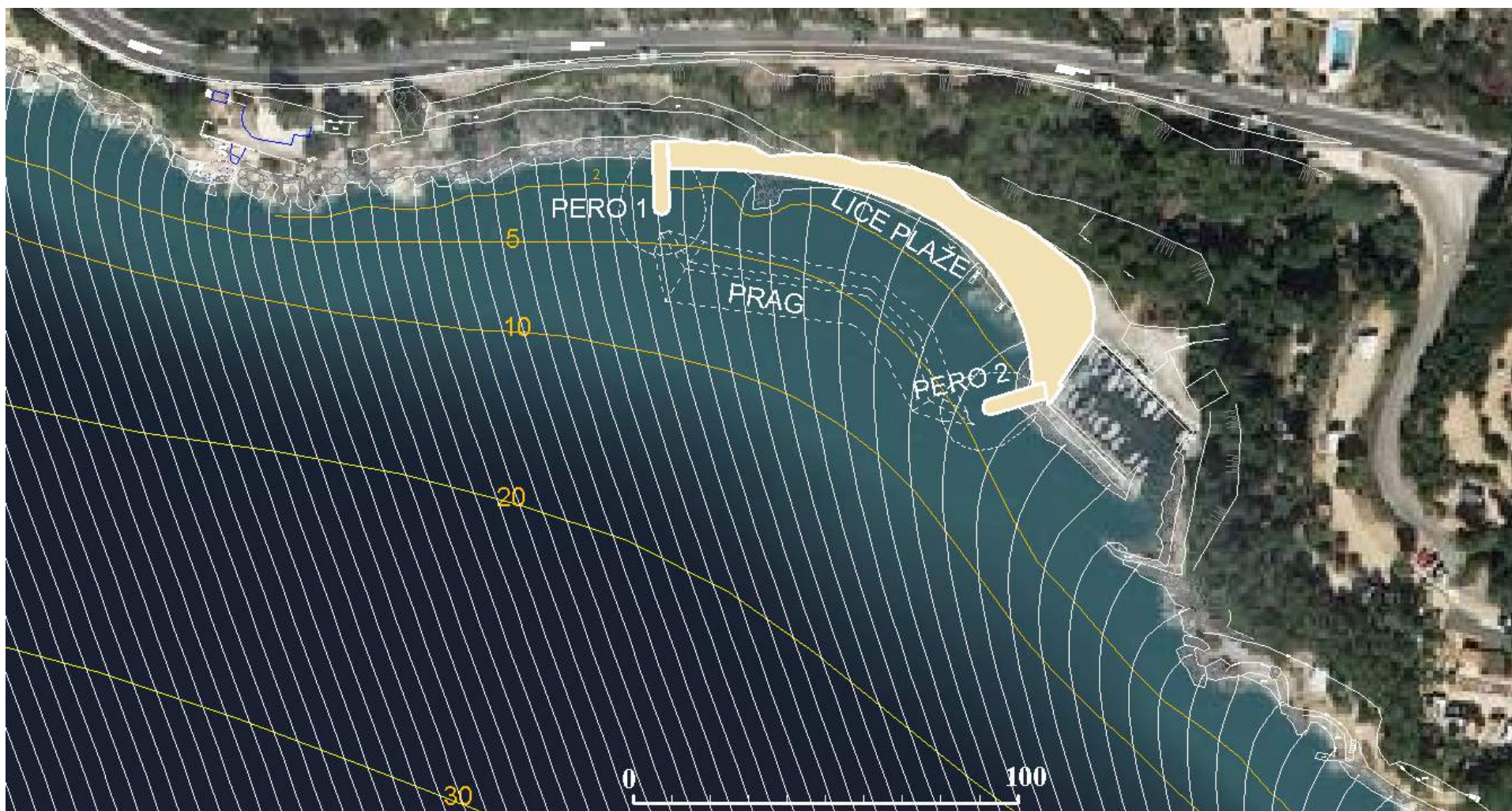
Slika 1.4. Djelovanje valova iz smjera SE
