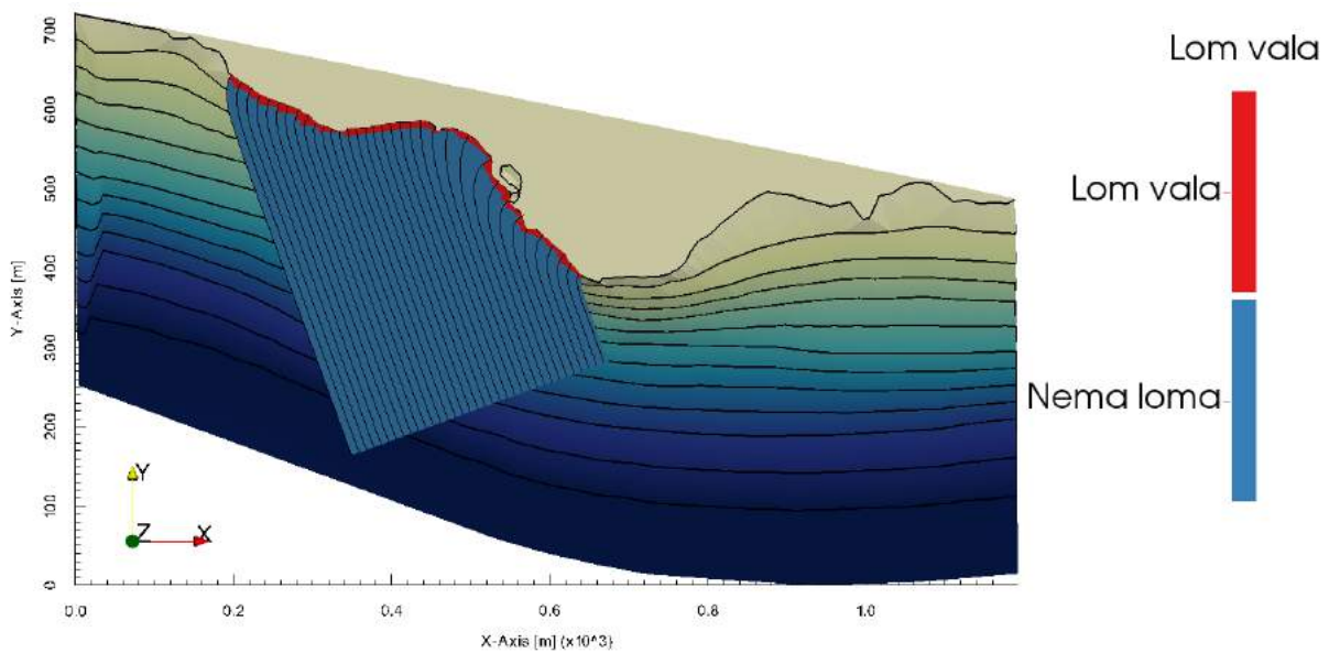
Slika 2.12. Detekcija loma vala za Sektor I - petogodišnji val ( H_s^5=2.12 m, T_0^5=5.40 s)
