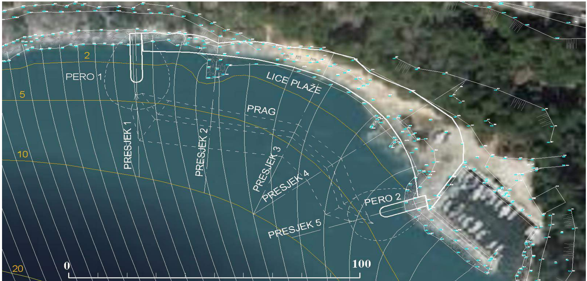
Slika 1.5. Rješenje rekonstrukcije i prihrane plaže
