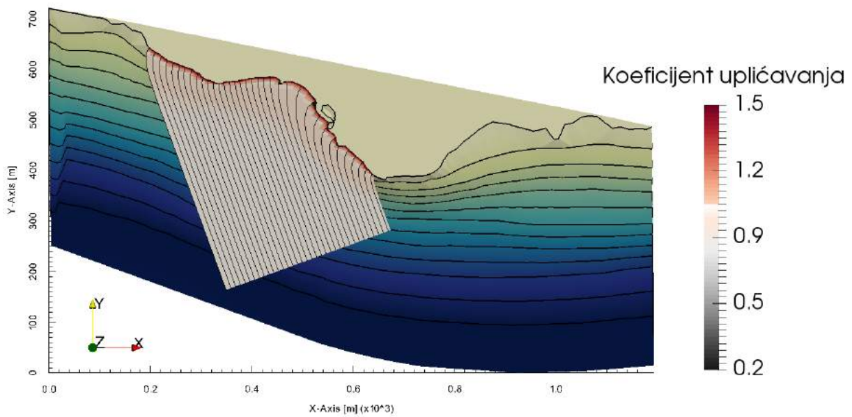
Slika 2.10. Utjecaj uplićavanja vala za Sektor I ( H_s^5=2.12 m, T_0^5=5.40 s)
