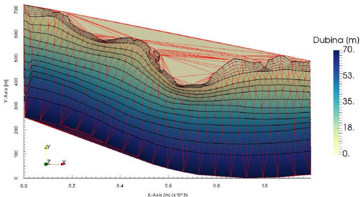
Slika 2.7. Mreža konačnih elemenata za akvatorij uvale Vojskovo
