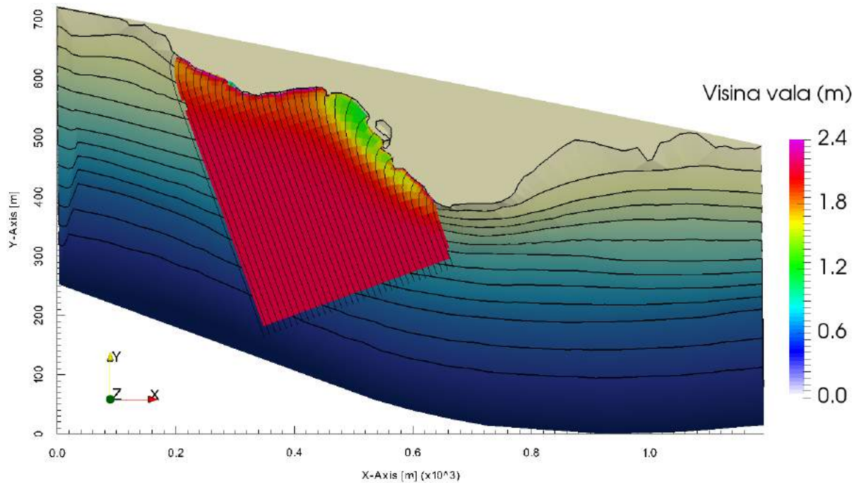
Slika 2.14. Polje značajnih visina vala za Sektor I ( H_s^5=2.12 m, T_0^5=5.40 s)
