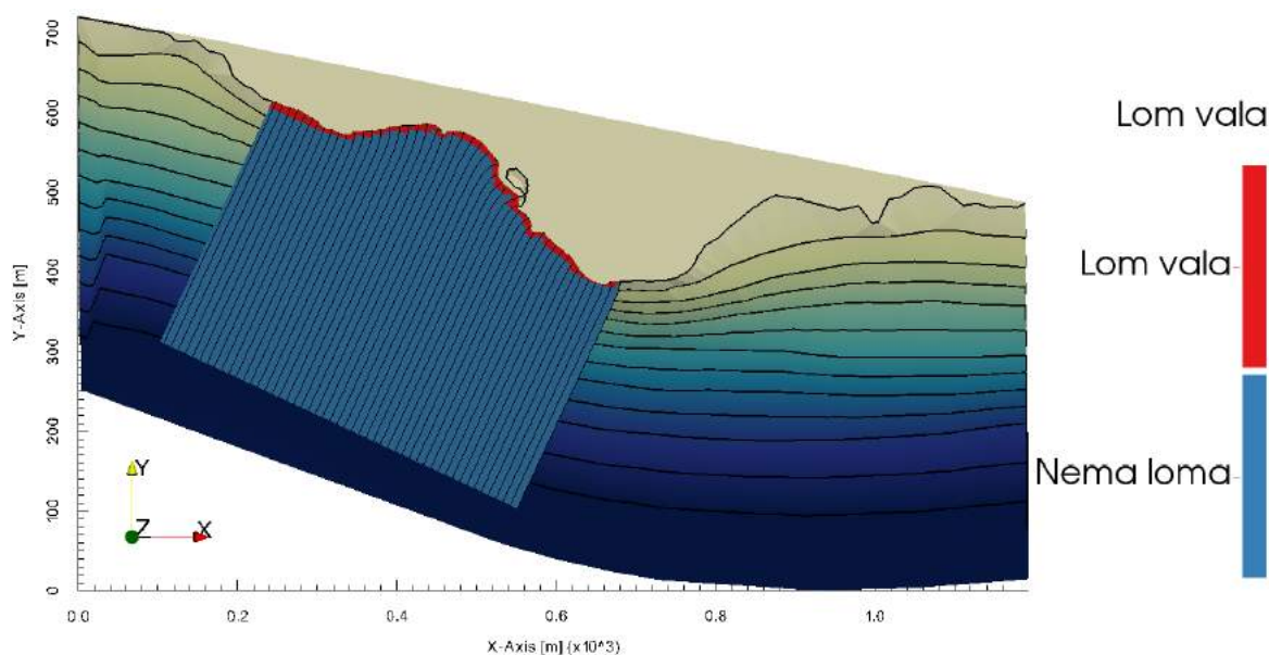
Slika 2.13. Detekcija loma vala za Sektor II - petogodišnji val ( H_s^5=1.73 m, T_0^5=4.88 s)
