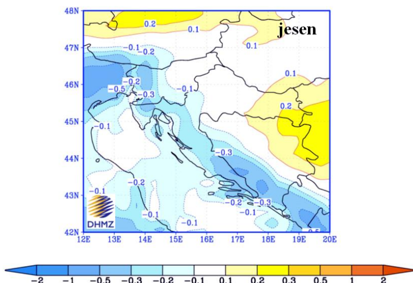
Slika 3.2.2.-3 Promjena oborine u Hrvatskoj (u mm/dan) u razdoblju 2011-2040. u odnosu na razdoblje 1961-1990. prema rezultatima srednjaka ansambla regionalnog klimatskog modela RegCM za A2 scenarij emisije plinova staklenika za jesen.
