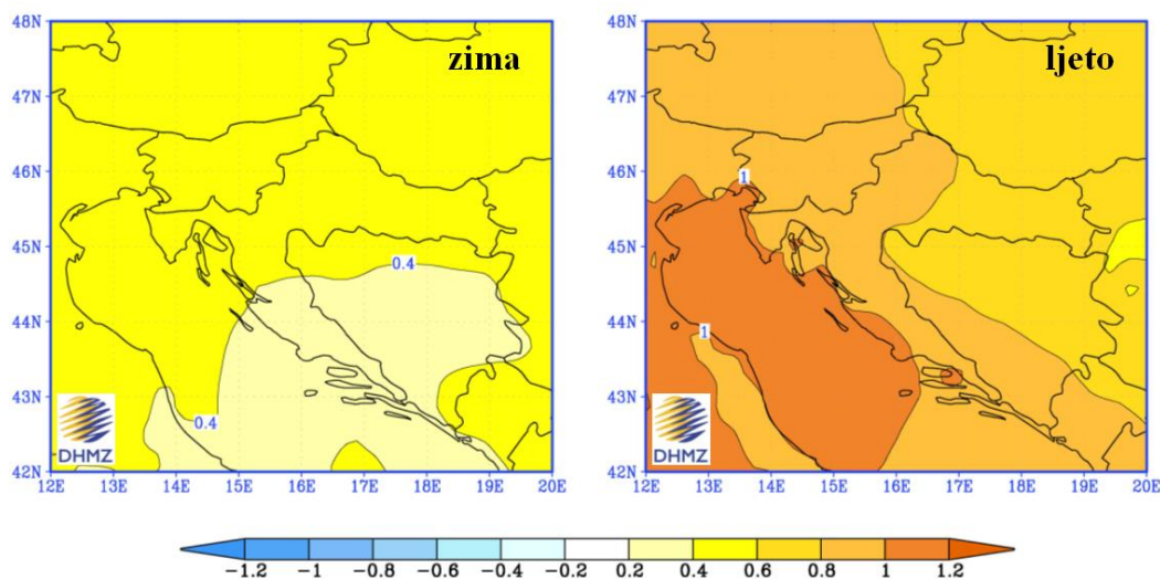
Slika 3.2.2.-1 Promjena prizemne temperature zraka (u ^{\circ}\text{C} ) u Hrvatskoj u razdoblju 2011-2040. u odnosu na razdoblje 1961-1990. prema rezultatima srednjaka ansambla regionalnog klimatskog modela RegCM za A2 scenarij emisije plinova staklenika za zimu (lijevo) i ljetno (desno).
