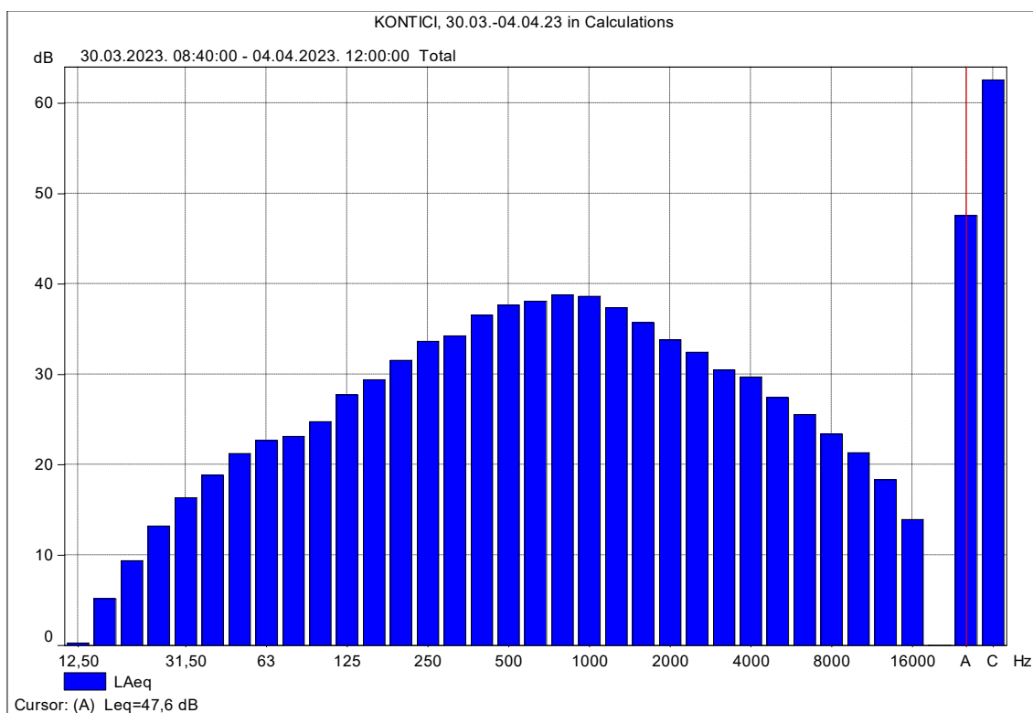
Slika 11 – Trećinskooktavni A-vrednovani spektar frekvencija – MM1 – 30.03.2023.- 04.04.2023.
