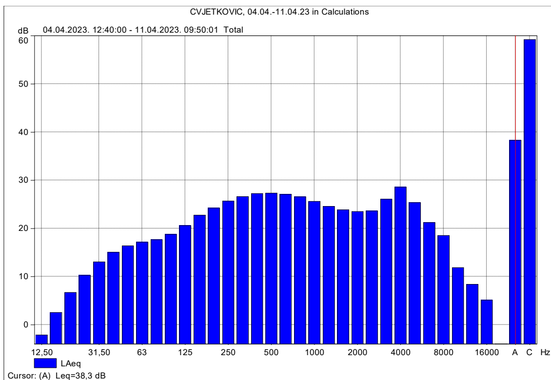
Slika 15 – Trećinskooktavni A-vrednovani spektar frekvencija – MM2 – 04.04.2023. - 11.04.2023.
