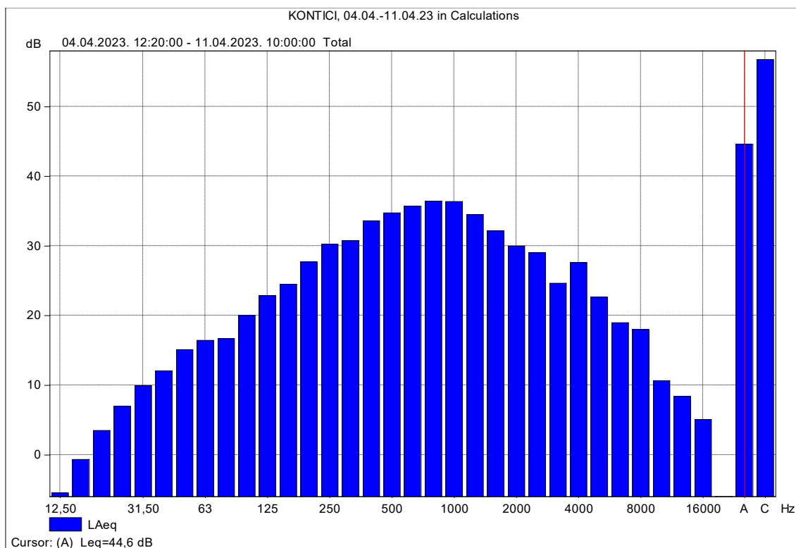
Slika 12 – Trećinskooktavni A-vrednovani spektar frekvencija – MM1 – 04.04.2023.- 11.04.2023.
