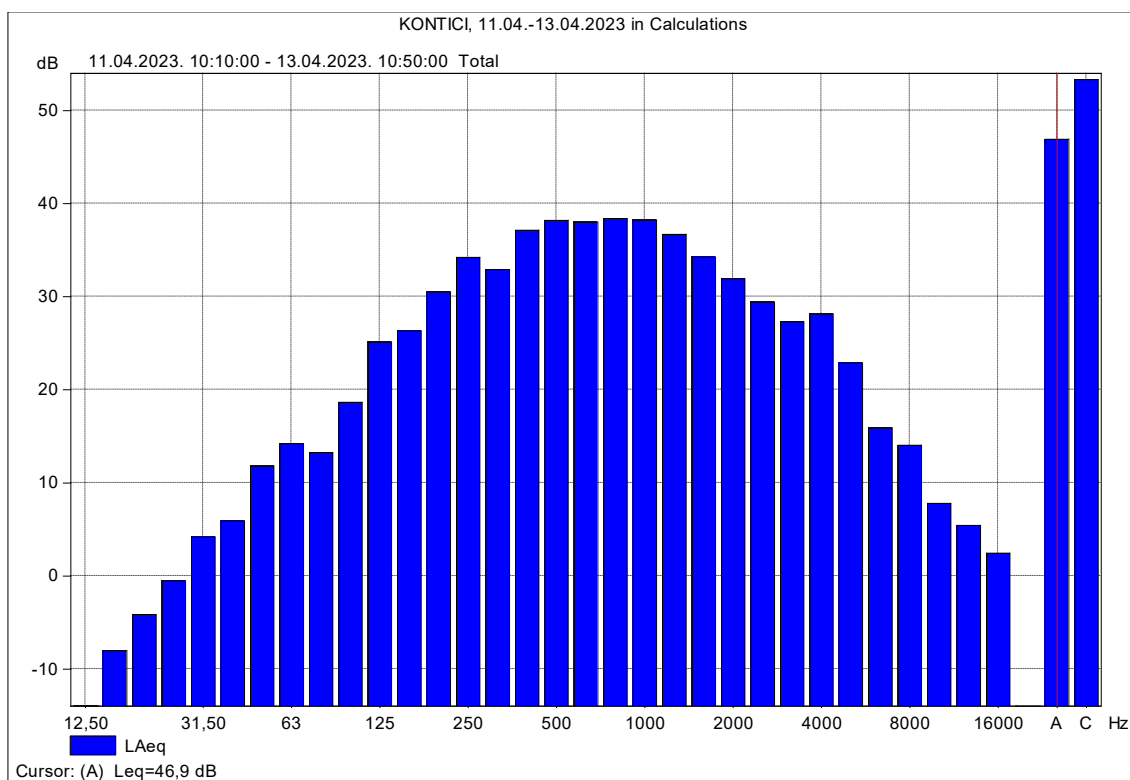
Slika 13 – Trećinskooktavni A-vrednovani spektar frekvencija – MM1 – 11.04.2023.- 13.04.2023.
