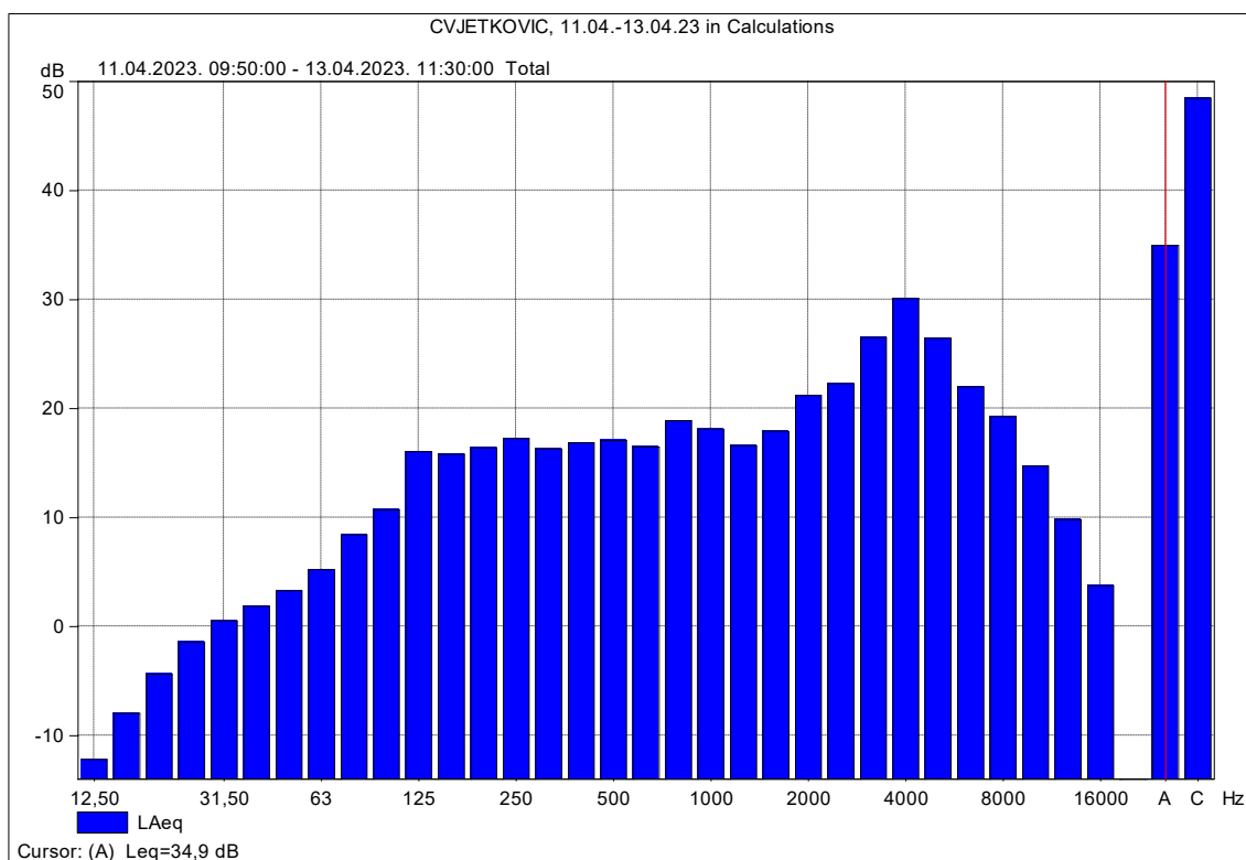
Slika 16 – Trećinskooktavni A-vrednovani spektar frekvencija – MM2 – 11.04.2023. - 13.04.2023.
