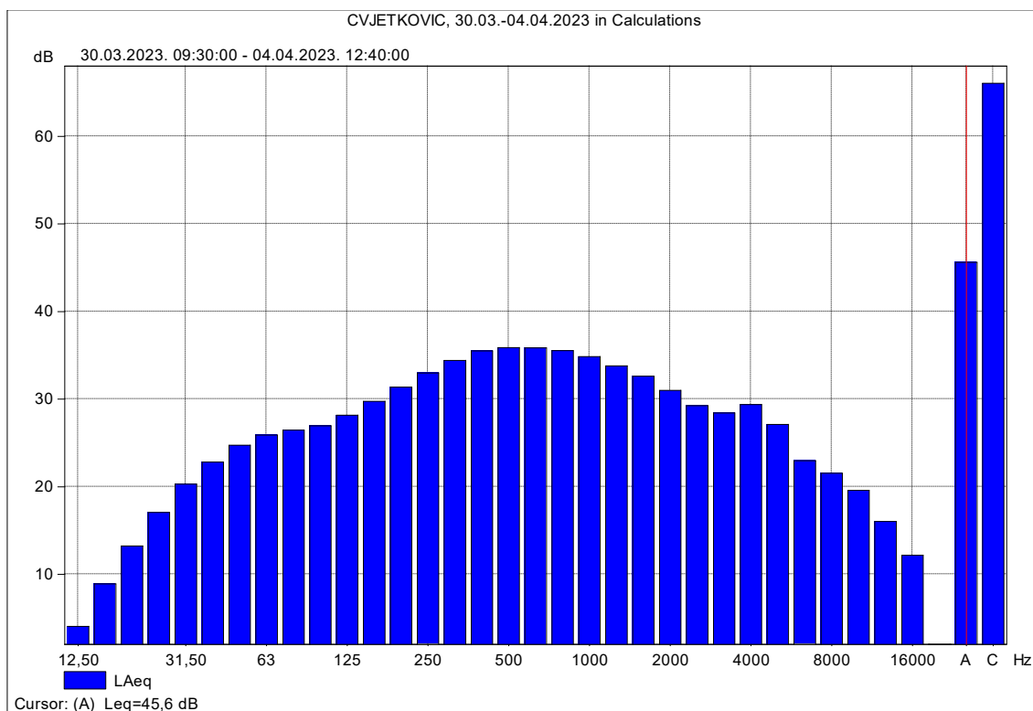
Slika 14 – Trećinskooktavni A-vrednovani spektar frekvencija – MM2 – 30.03.2023.- 04.04.2023.
